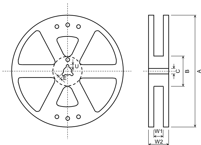
図 3.6.1 リール形状
