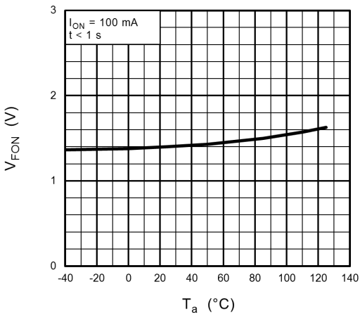
図 12.5 V_{FON} - T_a
