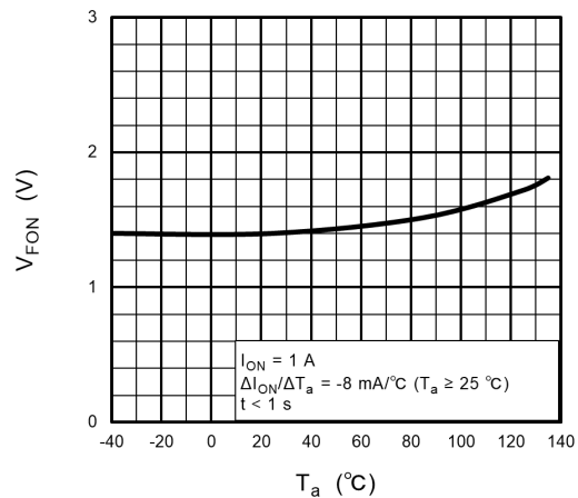
Fig. 12.6 V_{FON} - T_a
