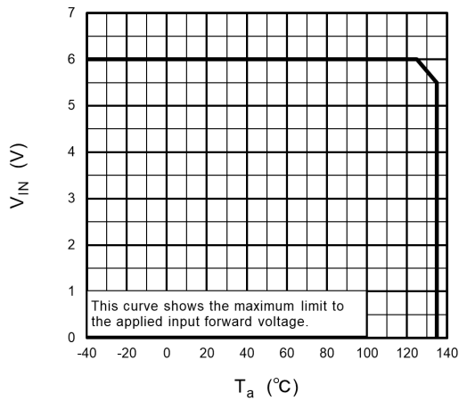
Fig. 12.1 V_{IN} - T_a
