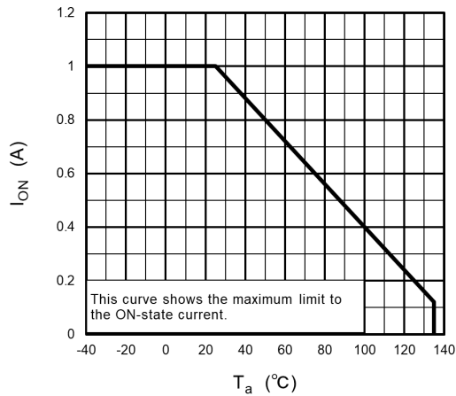
Fig. 12.3 I_{ON} - T_a
