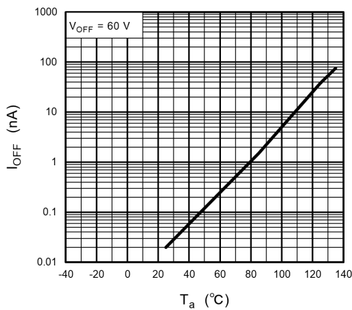
Fig. 12.11 I_{OFF} - T_a
