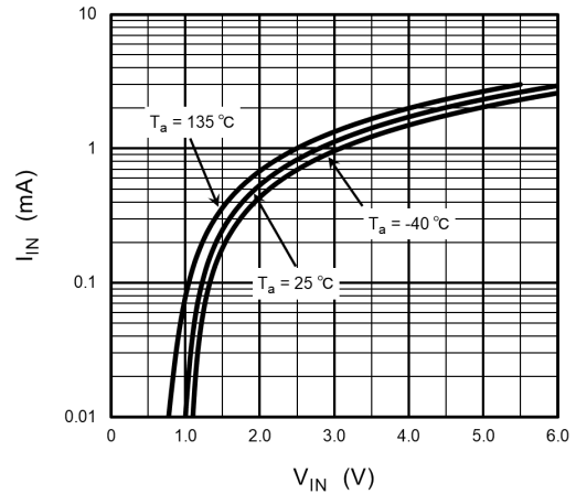
Fig. 12.2 I_{IN} - V_{IN}
