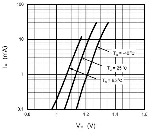
図 12.3 I_F - V_F
