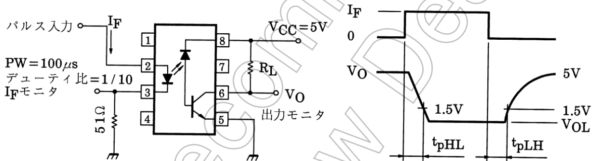
図1 伝達遅延時間測定回路、波形
