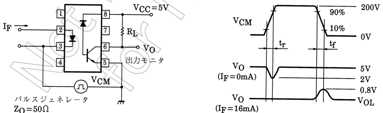
図2 コモンモードノイズ除去電圧測定回路、波形
