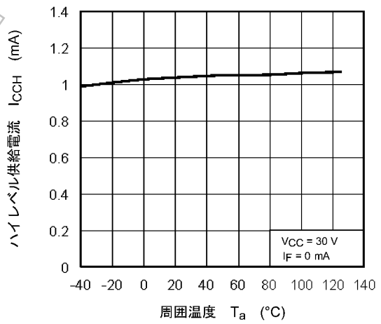
図 12.2.6 I_{CCH} - T_a
