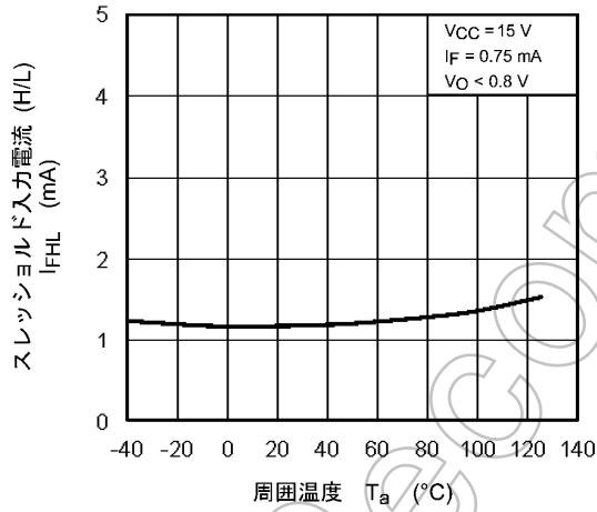
図 12.2.3 I_{FHL} - T_a
