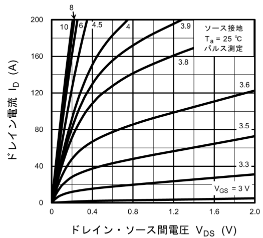
図 8.2 I_D - V_{DS}
