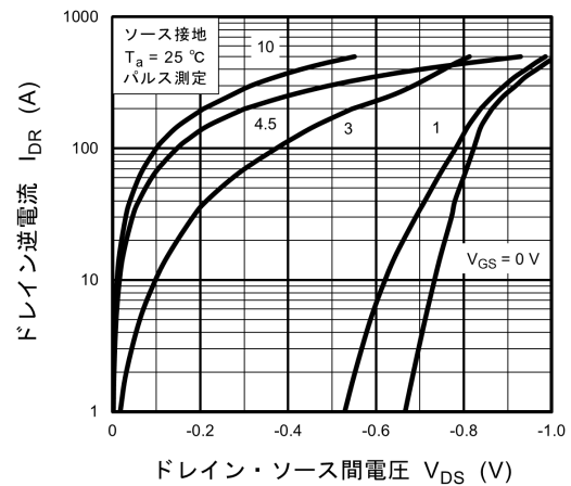
図 8.6 I_{DR} - V_{DS}
