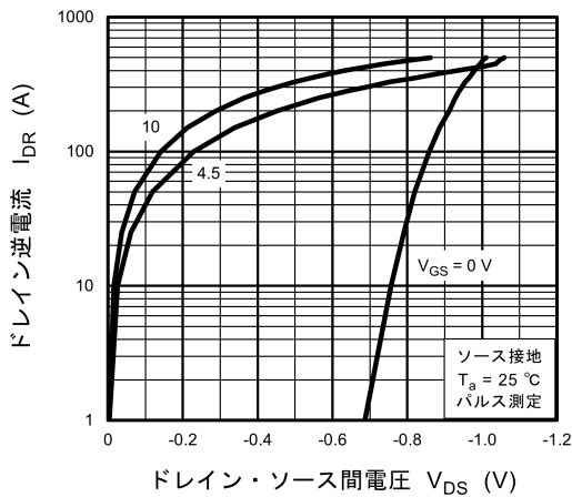
図 8.5 I_{DR} - V_{DS}
