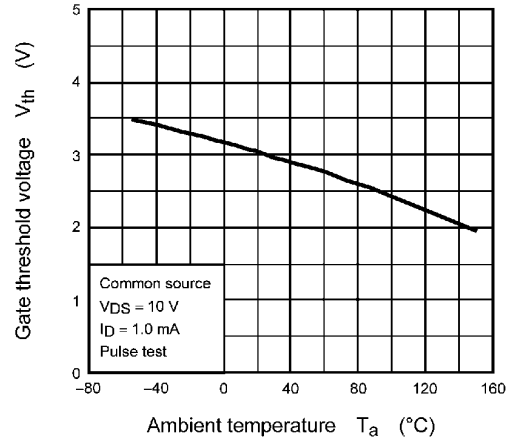
Fig. 8.8 V_{th} - T_a
