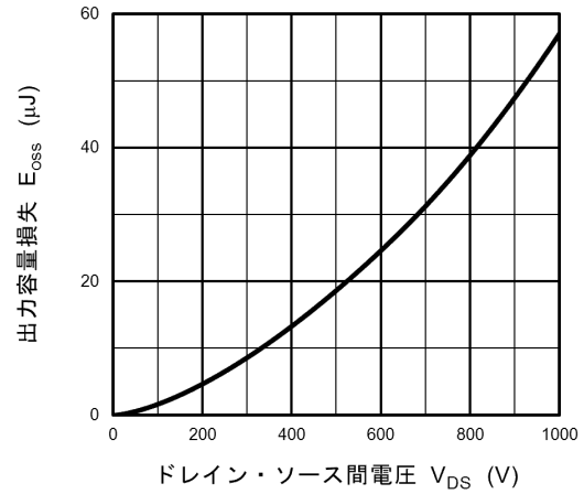
図 8.14 E_{oss} - V_{DS}
