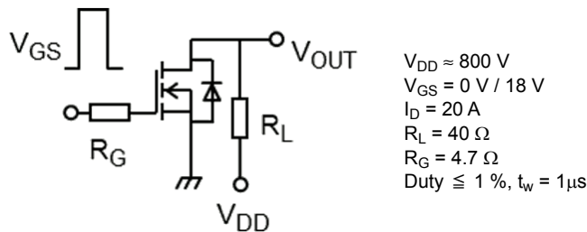
図 6.2.1 スwitchング時間の測定回路
