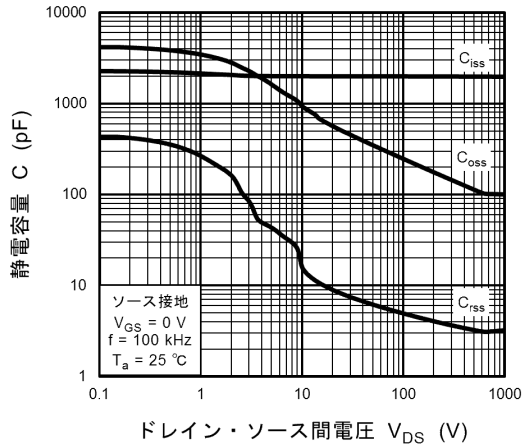
図 8.13 C - V_{DS}
