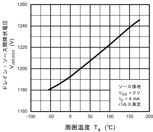
図 8.11 V_{DSS} - T_a
