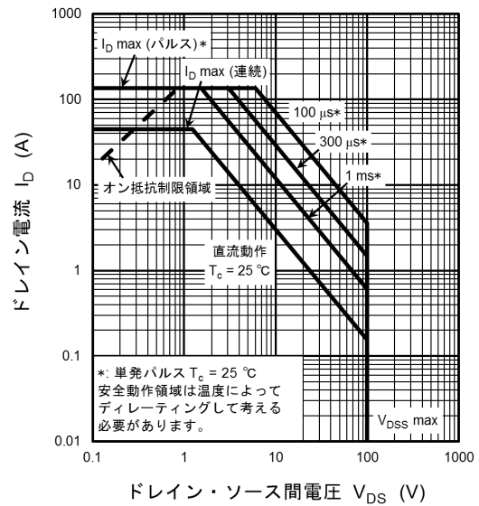
図 8.19 安全動作領域 (最大値 (保証値))
