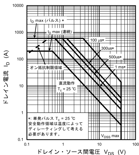
図 8.16 安全動作領域 (最大値 (保証値))
