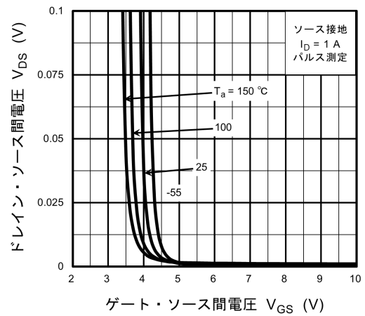
図 8.6 V_{DS} - V_{GS}
