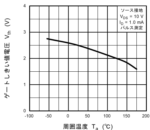
図 8.12 V_{th} - T_a
