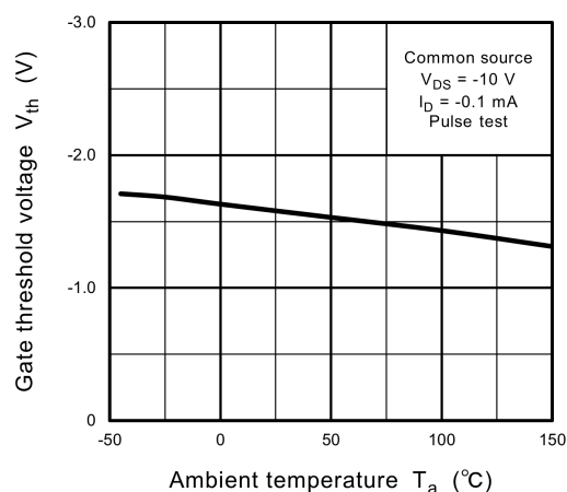
Fig. 9.6 V_{th} - T_a
