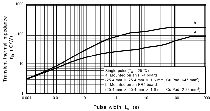
Fig. 9.9 r_{th} - t_w
