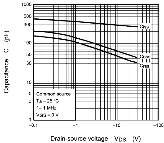
Fig. 9.7 C - V_{DS}
