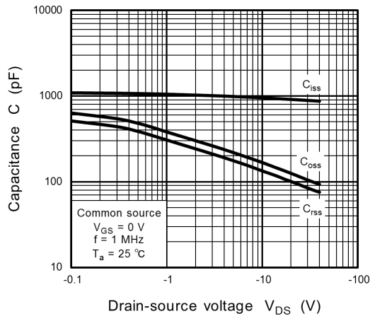
Fig. 8.7 C - V_{DS}
