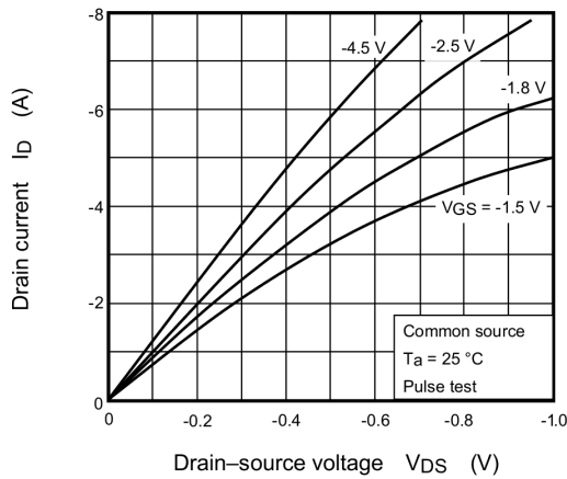
Fig. 8.1 I_D - V_{DS}
