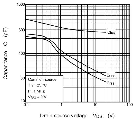
Fig. 8.7 C - V_{DS}
