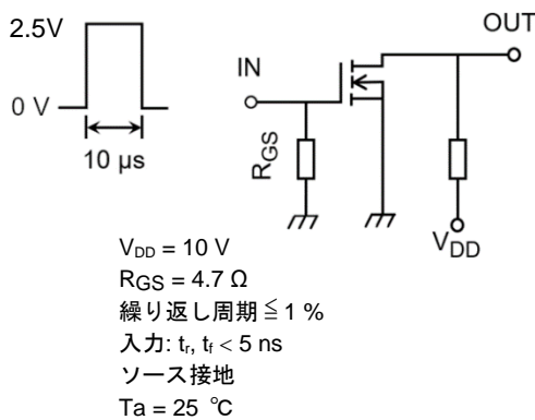
(a) 測定回路
