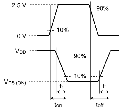
(c) 出力波形
