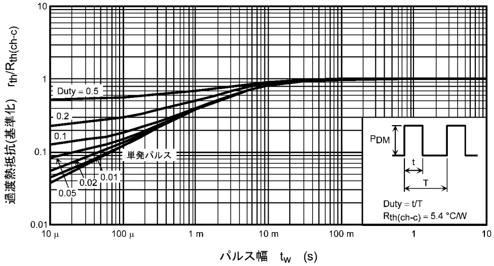
図 8.11 r_{th}/R_{th(ch-c)} - t_w (最大値 (保証値))
