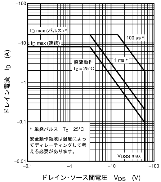
図 8.13 安全動作領域 (最大値 (保証値))
