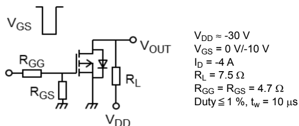
図 6.2.1 スwitching時間の測定回路
