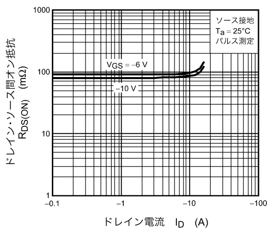
図 8.5 R_{DS(ON)} - I_D
