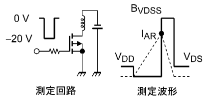
図 8.15 測定回路/測定波形
