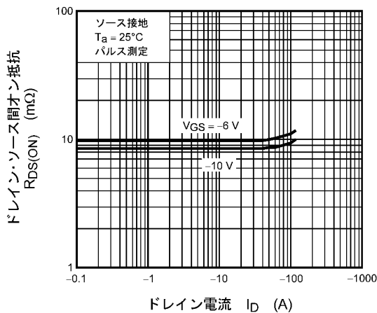
図 8.5 R_{DS(ON)} - I_D
