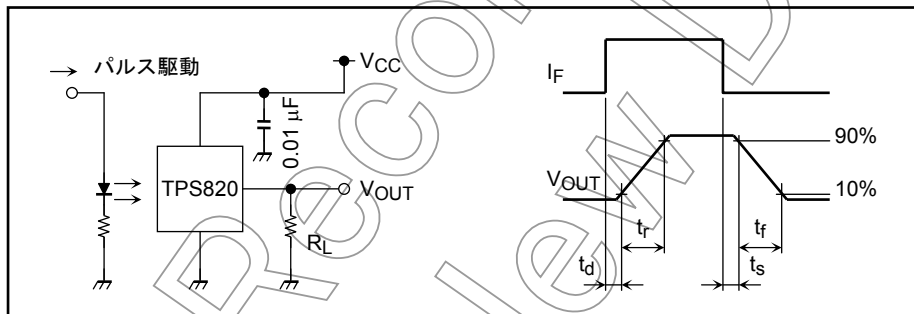
スイッチング時間測定回路、波形
