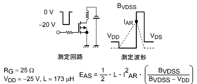
図 8.15 測定回路/測定波形
