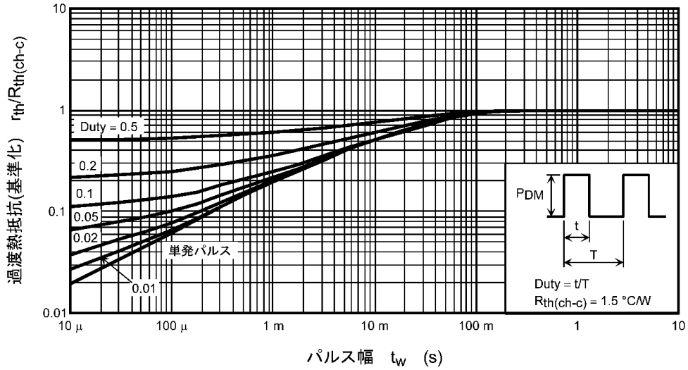
図 8.11 r_{th}/R_{th(ch-c)} - t_w (最大値 (保証値))
