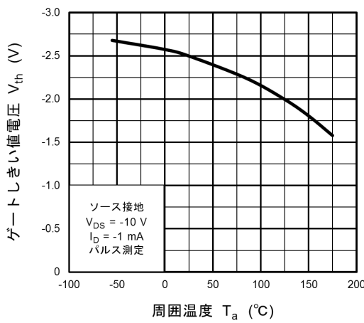
図 8.9 V_{th} - T_a
