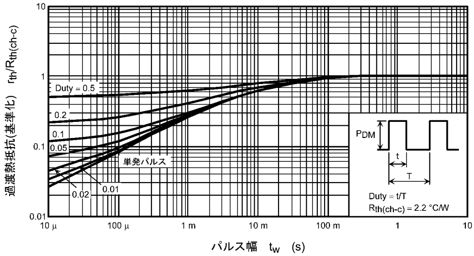
図 8.11 r_{tr}/R_{th(ch-c)} - t_w (最大値 (保証値))
