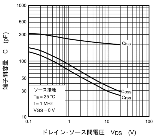
図 7.9 C - V_{DS}
