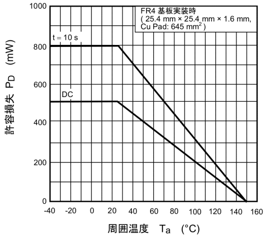
図 7.13 P_D - T_a
