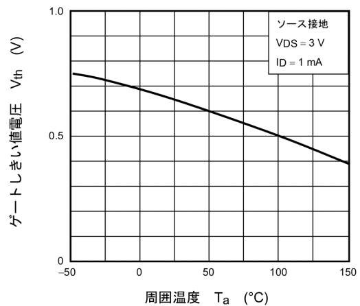
図 7.6 V_{th} - T_a
