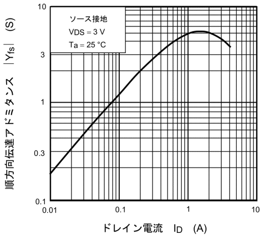
図 7.7 |Y_{fs}| - I_D
