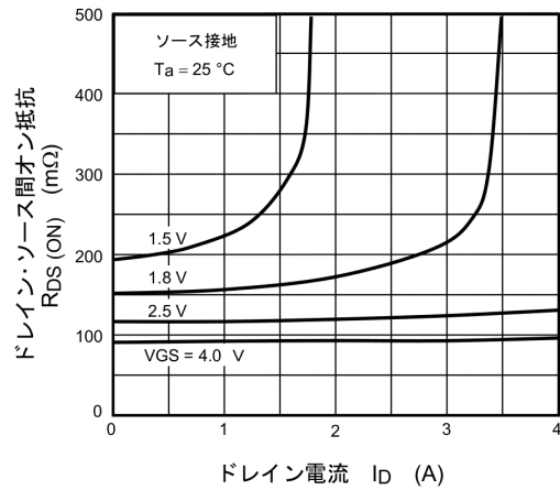
図 7.4 R_{DS(ON)} - I_D
