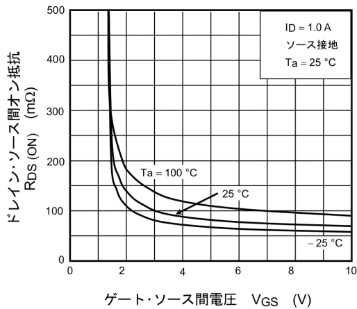
図 7.3 R_{DS(ON)} - V_{GS}
