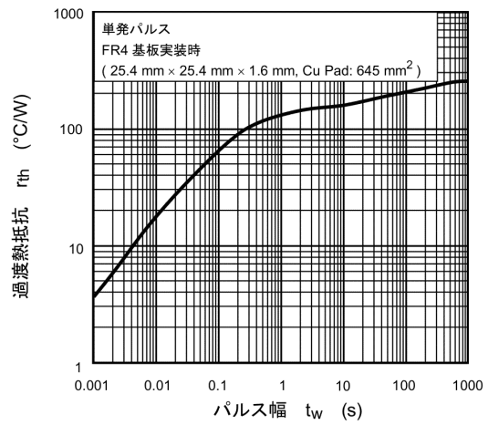
図 7.12 r_{th} - t_w
