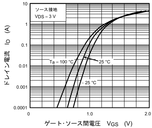
図 7.2 I_D - V_{GS}
