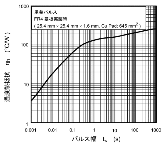
図 7.12 r_{th} - t_w
