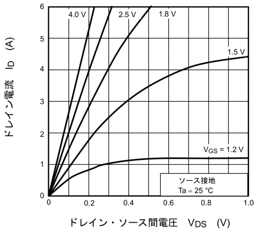
図 7.1 I_D - V_{DS}
