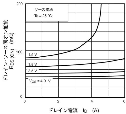
図 7.4 R_{DS(ON)} - I_D
