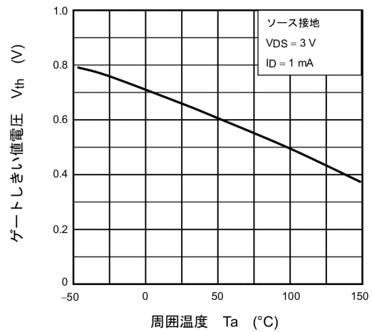
図 7.6 V_{th} - T_a
