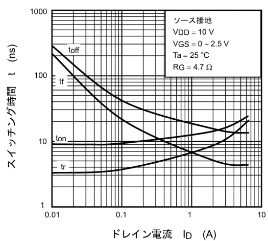
図 7.10 t - I_D
