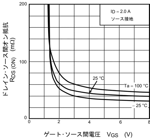
図 7.3 R_{DS(ON)} - V_{GS}
