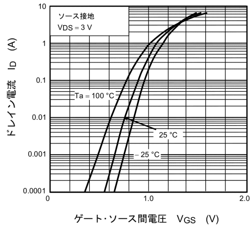
図 7.2 I_D - V_{GS}
