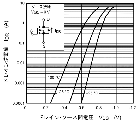
図 7.8 I_{DR} - V_{DS}
