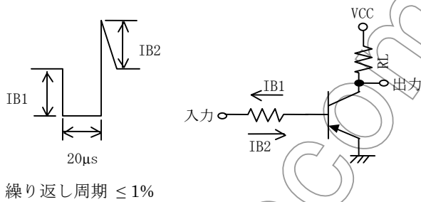
図1.スイッチング時間測定回路
