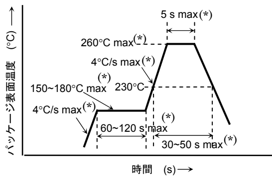
Pbフリーはんだ時の温度プロフィール例
