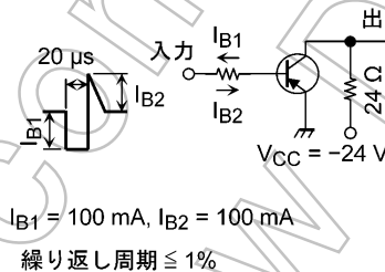
図 5.2.1 スwitching時間の測定回路
