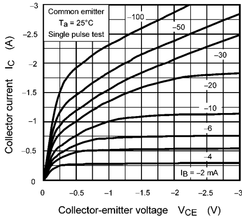
Fig. 7.1 I_C - V_{CE}
