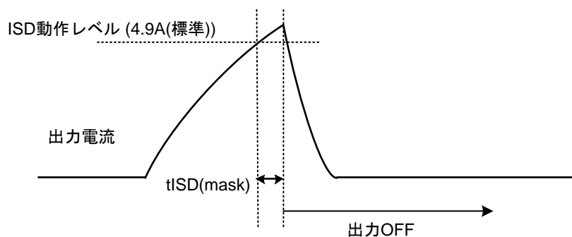
図 8-1 TB67H450AFNG の ISD 動作
