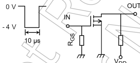
図 5.3.1 スwitchング時間の測定回路
