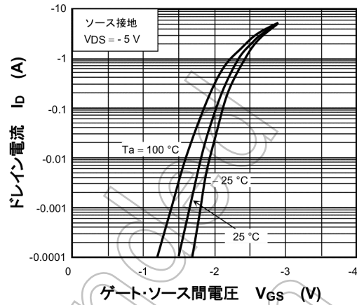
図 7.2 I_D - V_{GS}
