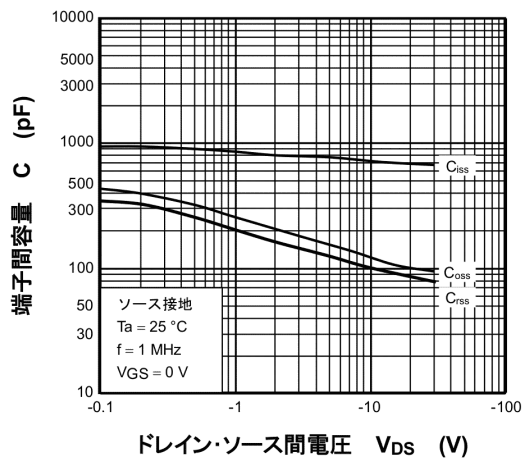
図 7.9 C - V_{DS}
