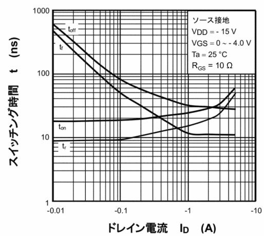
図 7.10 t - I_D
