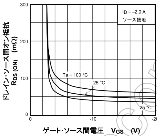
図 7.3 R_{DS(ON)} - V_{GS}
