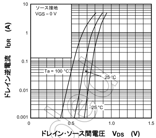
図 7.8 I_{DR} - V_{DS}
