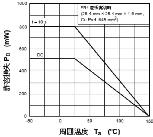
図 7.13 P_D - T_a
