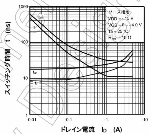
図 7.10 t - I_D
