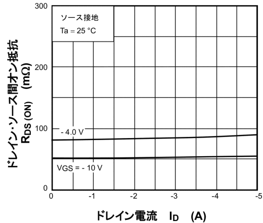
図 7.4 R_{DS(ON)} - I_D
