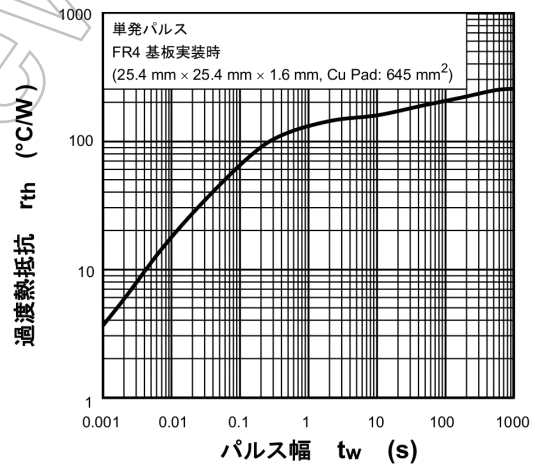
図 7.12 r_{th} - t_w
