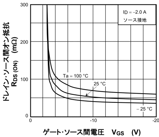
図 7.3 R_{DS(ON)} - V_{GS}
