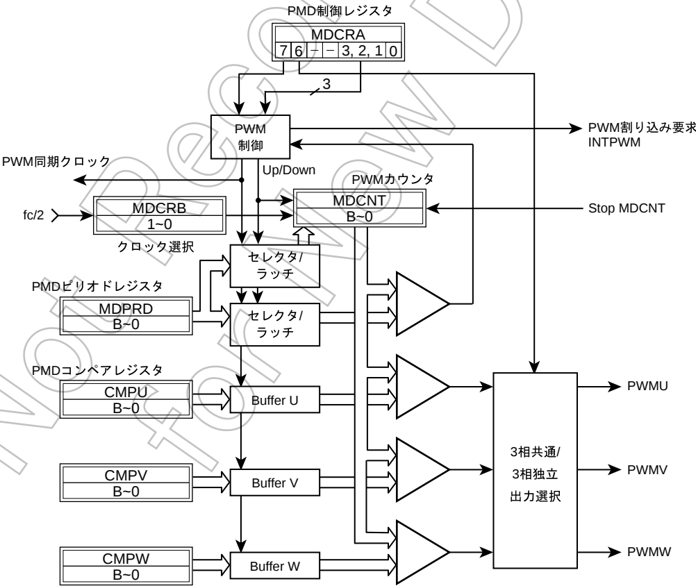
図 13-10 パルス幅変調回路
