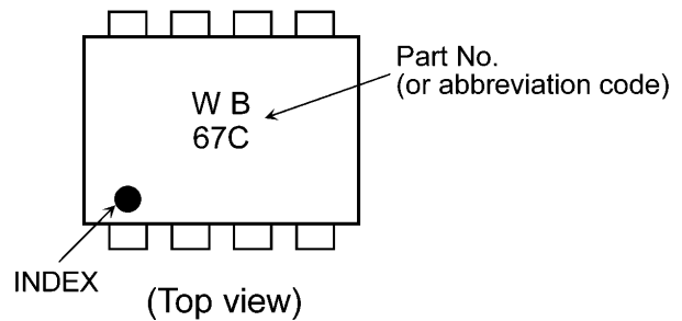
TC7WB67CFK
