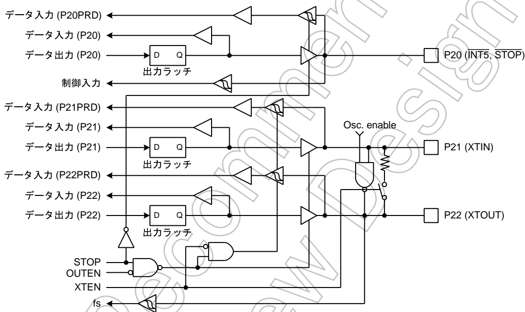
図 5-4 P2 ポート
