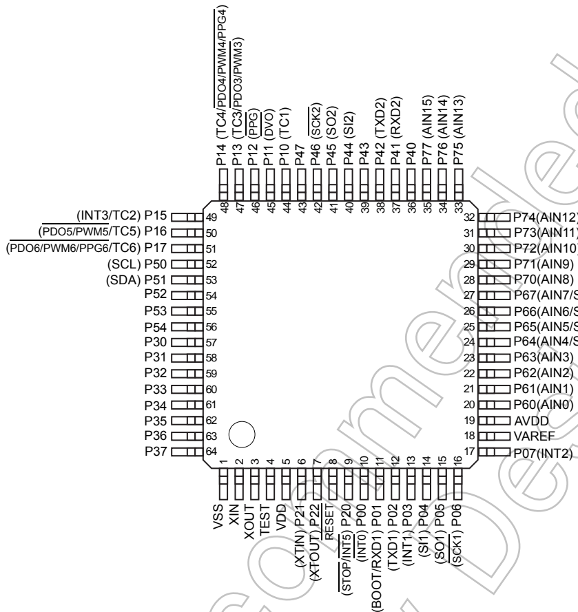
図 1-1 ピン配置図
