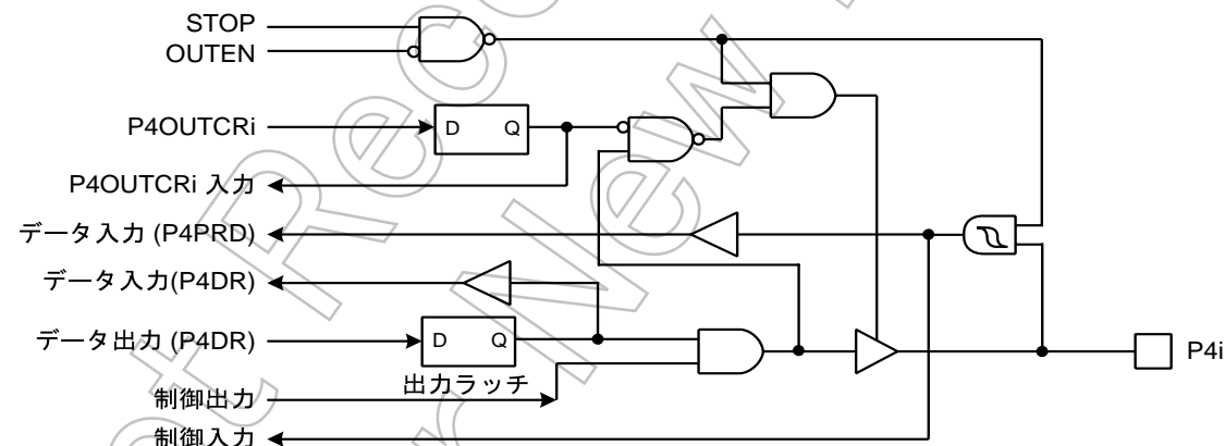
図 5-6 P4 ポート
