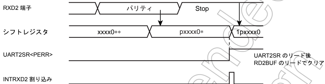
図 13-5 パリティエラーの発生
