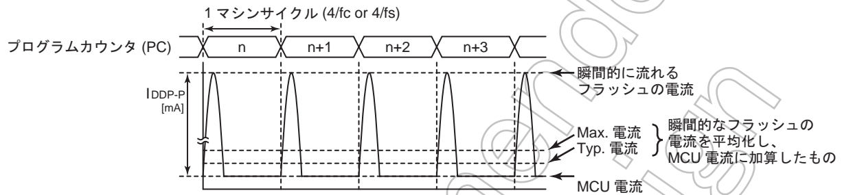
図 22-1 フラッシュメモリの間欠動作
