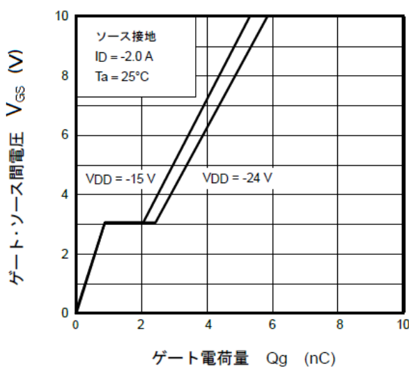
図 7.11 ダイナミック入力特性
