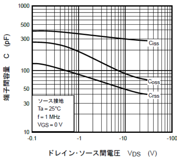
図 7.9 C - V_{DS}
