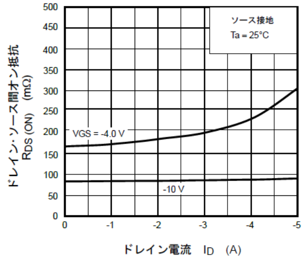
図 7.4 R_{DS(ON)} - I_D
