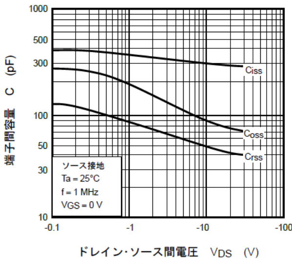
図 7.9 C - V_{DS}
