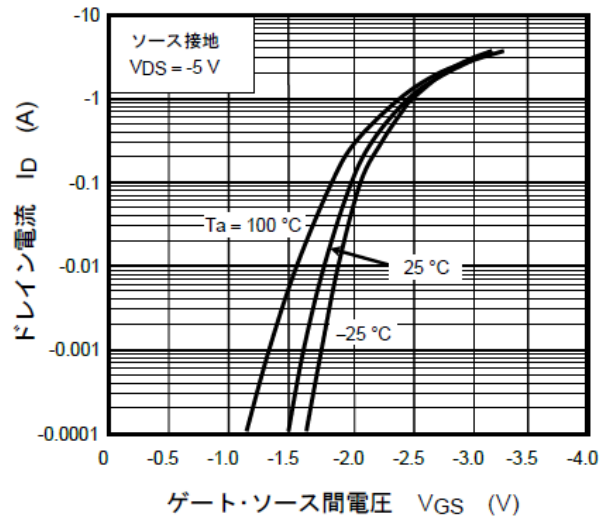
図 7.2 I_D - V_{GS}
