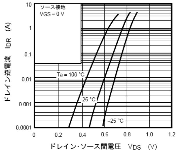
図 7.8 I_{DR} - V_{DS}
