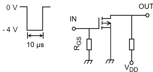
図 5.3.1 スイッチング時間の測定回路
