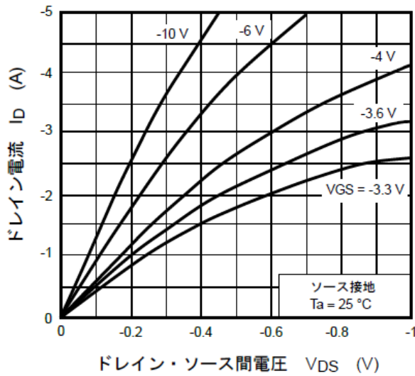
図 7.1 I_D - V_{DS}
