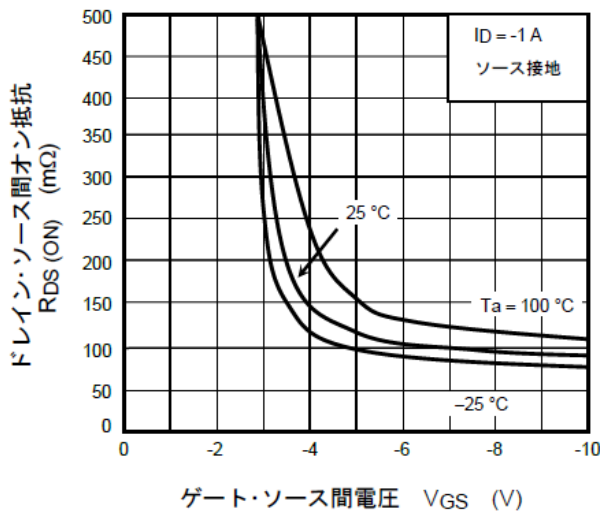
図 7.3 R_{DS(ON)} - V_{GS}
