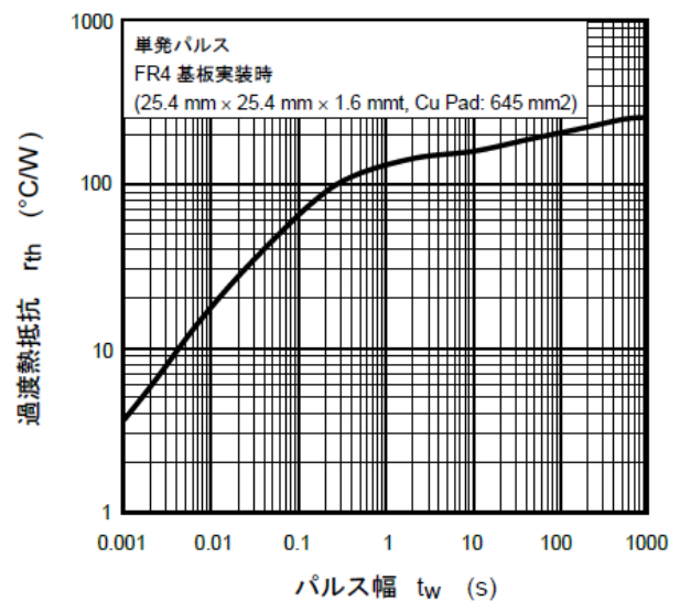
図 7.12 r_{th} - t_w
