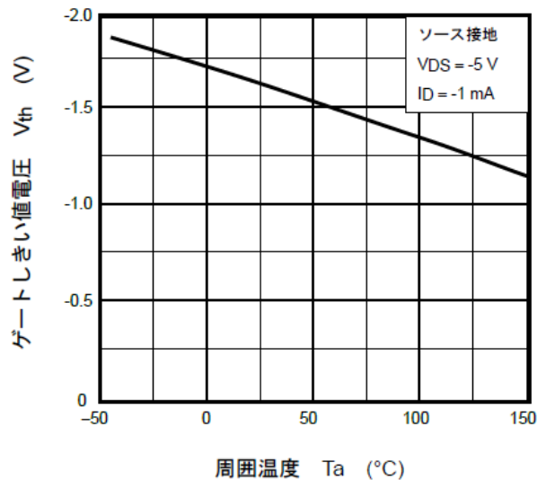
図 7.6 V_{th} - T_a
