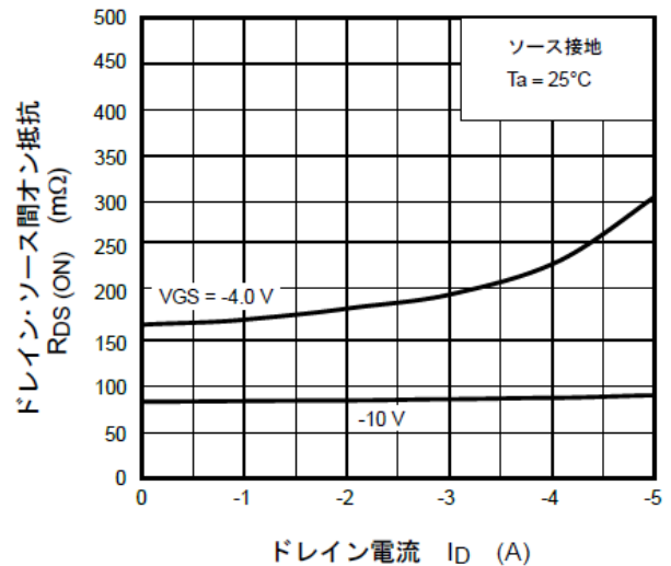
図 7.4 R_{DS(ON)} - I_D
