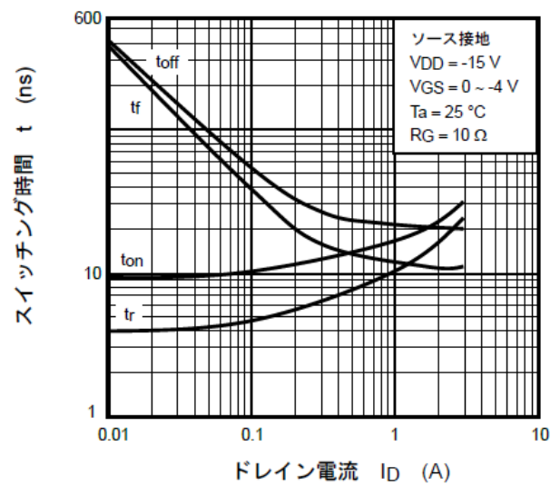
図 7.10 t - I_D
