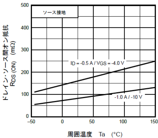
図 7.5 R_{DS(ON)} - T_a
