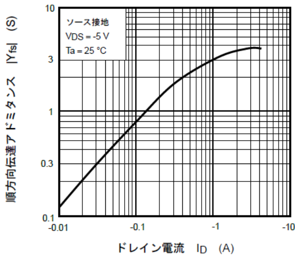
図 7.7 |Y_{fs}| - I_D
