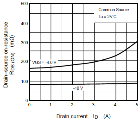
Fig. 7.4 R_{DS(ON)} - I_D
