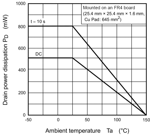
Fig. 7.13 P_D - T_a
