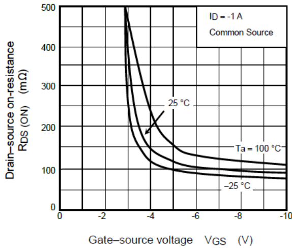
Fig. 7.3 R_{DS(ON)} - V_{GS}
