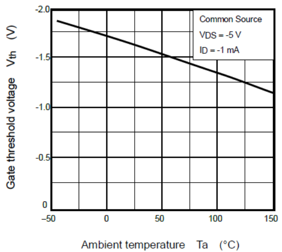
Fig. 7.6 V_{th} - T_a
