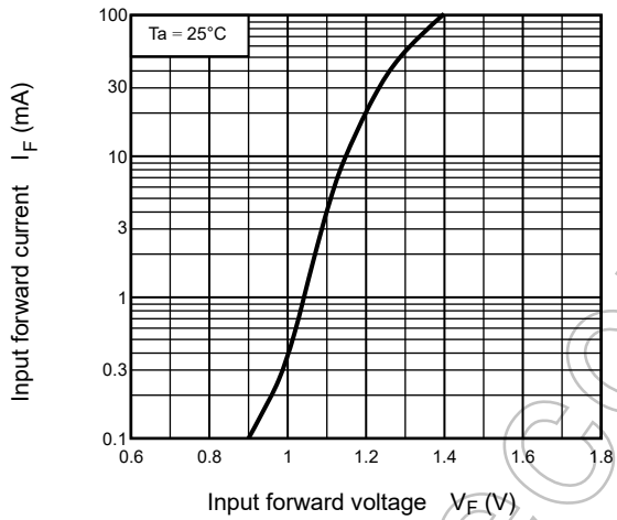
Fig.12.3 I_F - V_F
