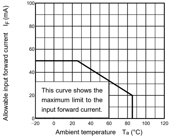
Fig.12.1 I_F - T_a
