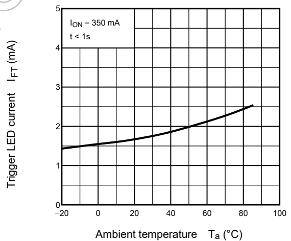
Fig.12.6 I_{FT} - T_a
