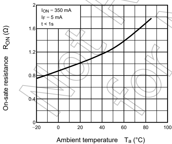
Fig.12.5 R_{ON} - T_a
