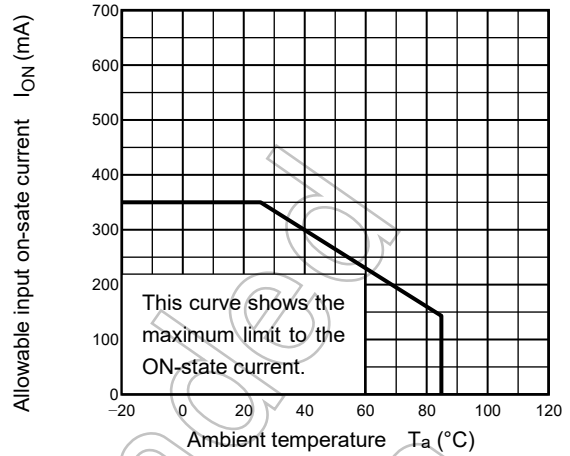
Fig.12.2 I_{ON} - T_a
