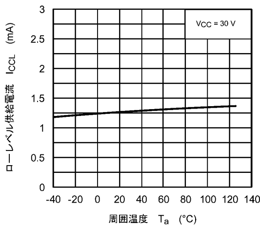
図 13.2.5 I_{CCL} - T_a
