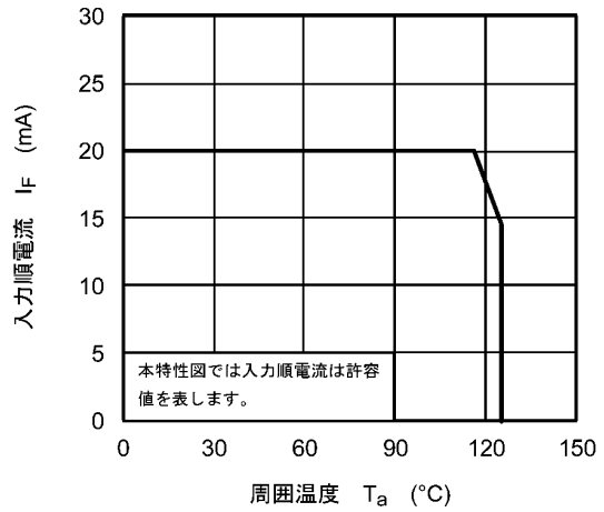
図 13.2.2 I_F - T_a
