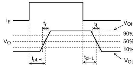
図 13.1.7 伝搬遅延時間測定回路, 波形
