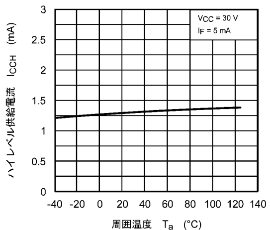
図 13.2.6 I_{CCH} - T_a
