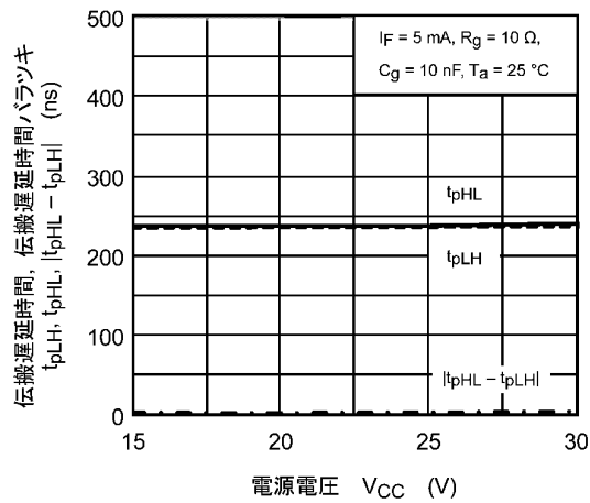
図 13.2.15 t_{pHL} , t_{pLH} , |t_{pHL} - t_{pLH}| - V_{CC}
