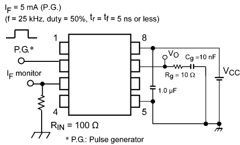
図 13.1.7 伝搬遅延時間測定回路, 波形
