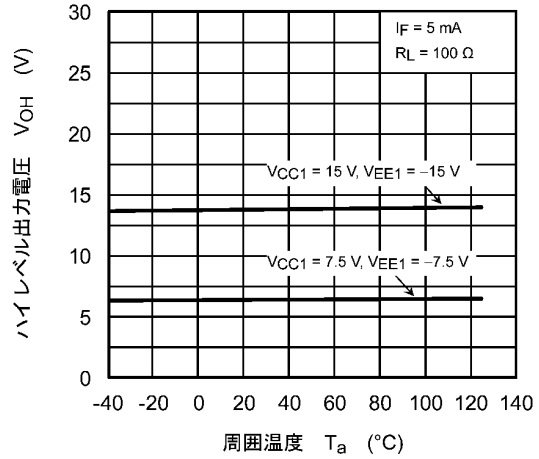
図 13.2.8 VOH - Ta
