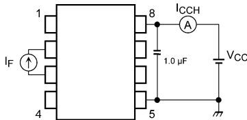
図 13.1.5 I CCH 測定回路
