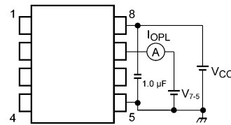
図 13.1.2 I OPL 測定回路
