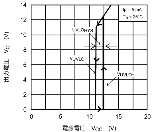
図 13.2.12 VO(VUVLO) - VCC
