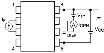
図 13.1.1 I OPH 測定回路
