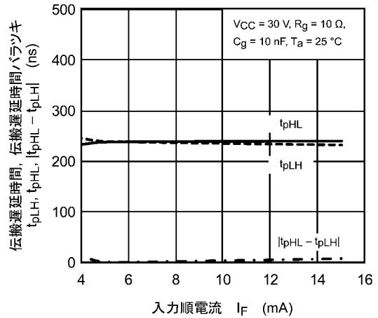
図 13.2.14 t_{pHL} , t_{pLH} , |t_{pHL} - t_{pLH}| - I_F
