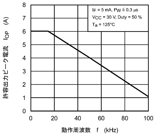
図 13.2.11 IOP - f
