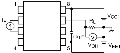
図 13.1.3 V OH 測定回路
