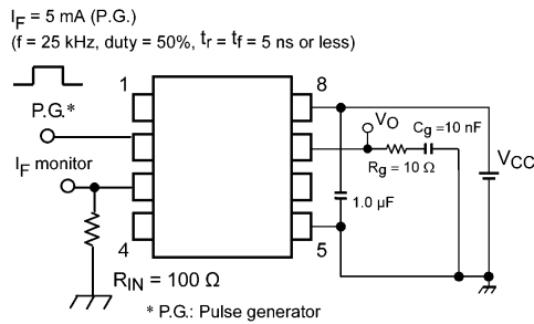
図 13.1.7 伝搬遅延時間測定回路, 波形
