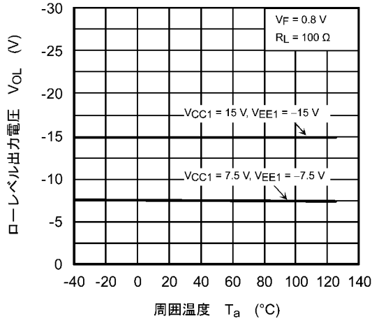
図 13.2.7 VOL - Ta
