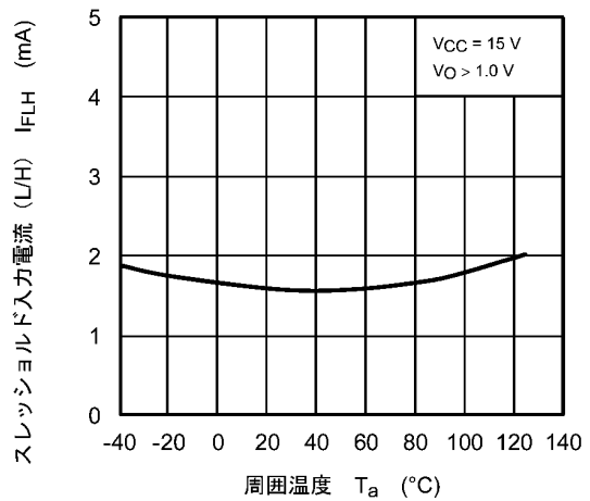
図 13.2.4 I_{FLH} - T_a
