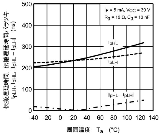
図 13.2.13 t_{pHL} , t_{pLH} , |t_{pHL} - t_{pLH}| - T_a
