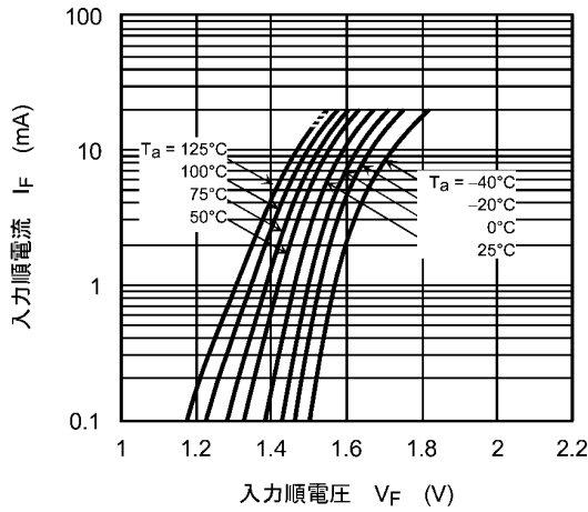
図 13.2.1 I_F - V_F
