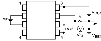
図 13.1.4 V OL 測定回路
