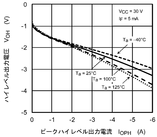
図 13.2.10 VOH - IOPH
