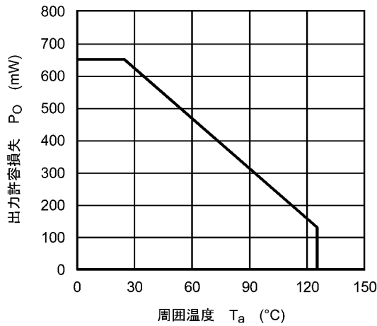
図 13.2.3 P_O - T_a
