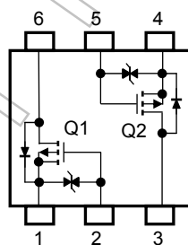
内部接続 (top view)
