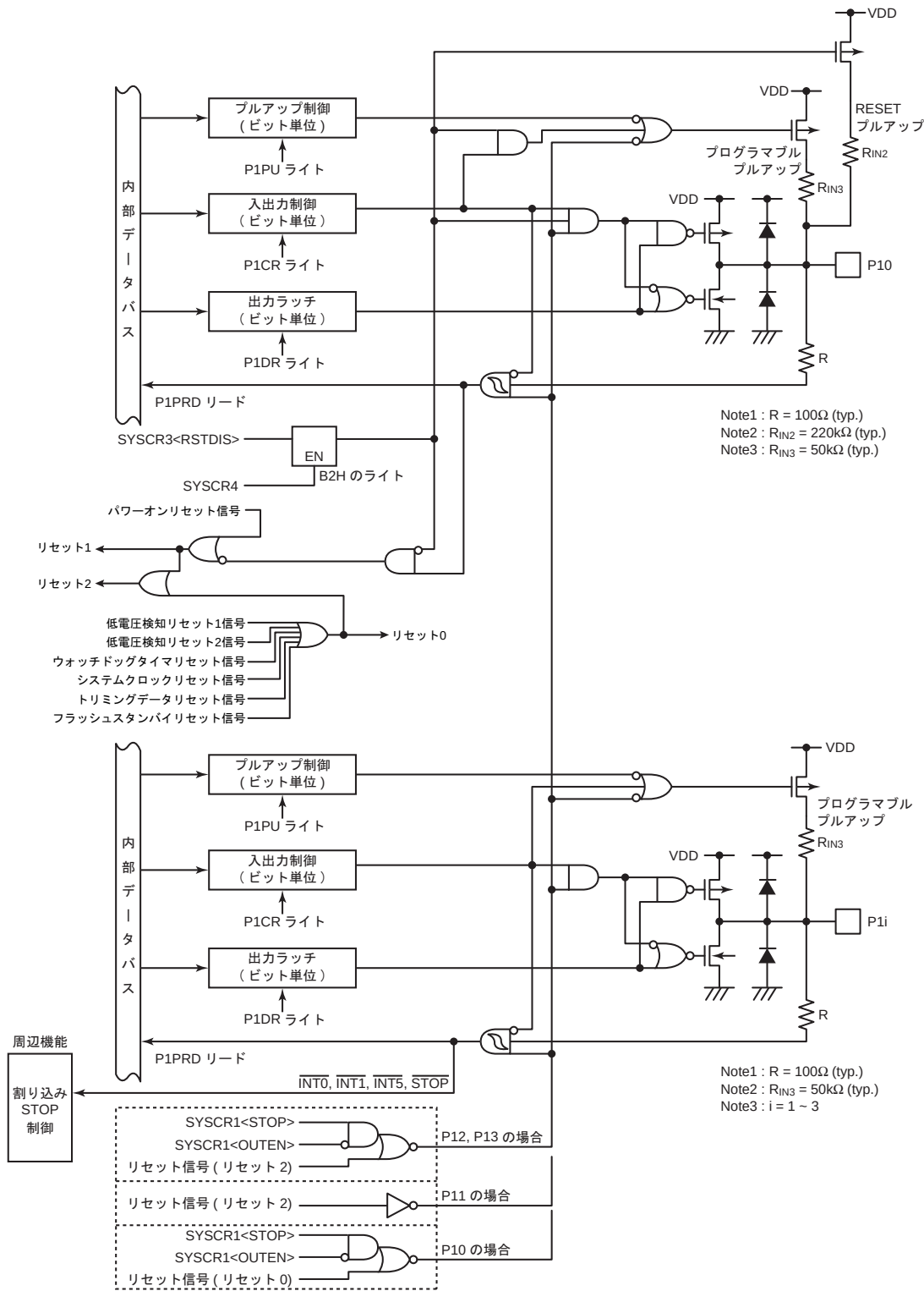
図 8-4 P1 ポート
