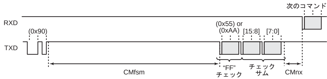
図 22-11 フラッシュメモリ SUM 出力コマンド
