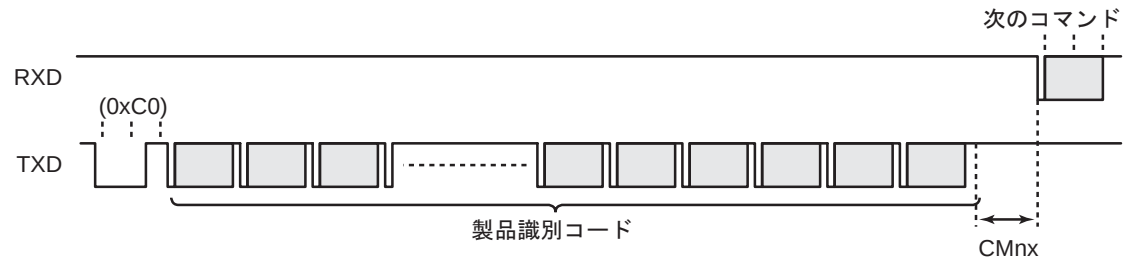
図 22-12 製品識別コード出力コマンド
