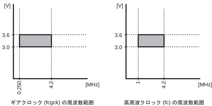
図 25-3 ギアクロック (fcgck) と 高周波クロック (fc)
