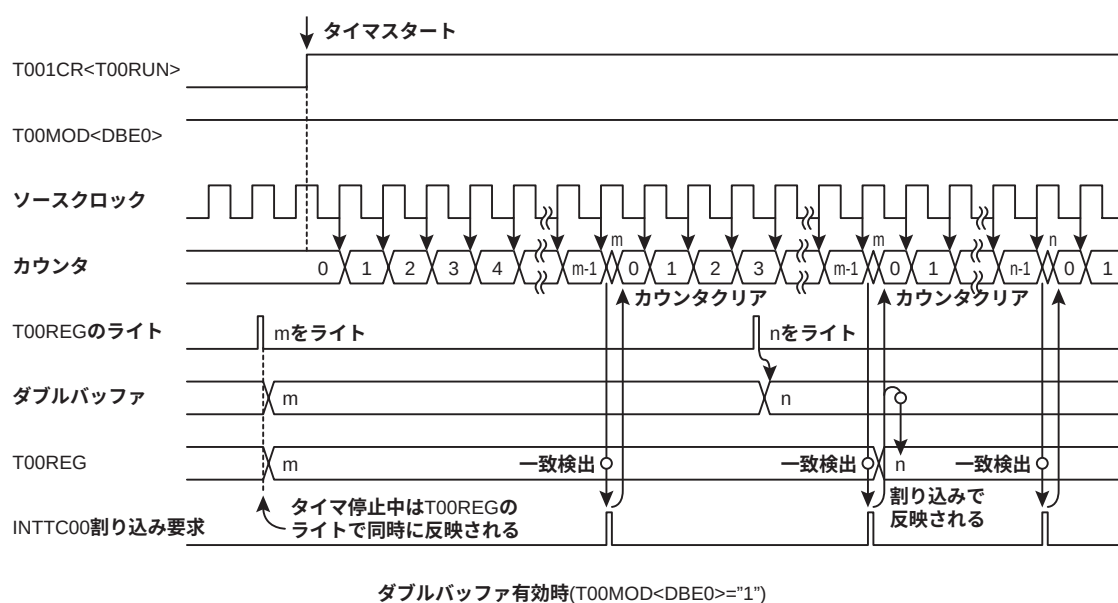
図 14-2 タイマモードタイミングチャート
