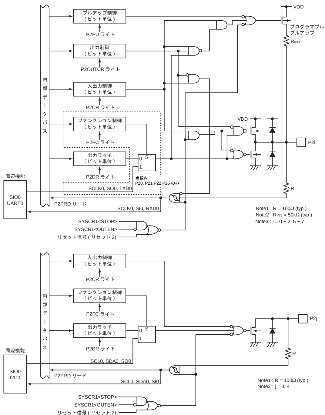
図 8-5 P2 ポート
