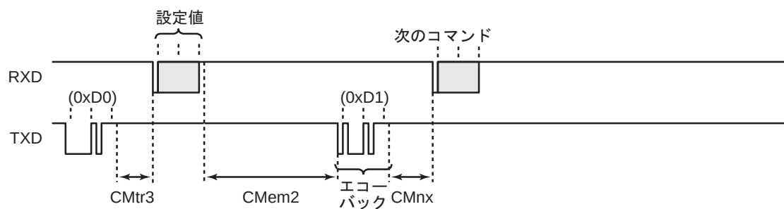
図 22-14 マスク ROM エミュレーション設定コマンド
