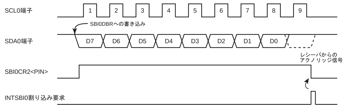
図 18-18 SBI0CR1<BC>=“000”，SBI0CR1<ACK>=“1” の場合
