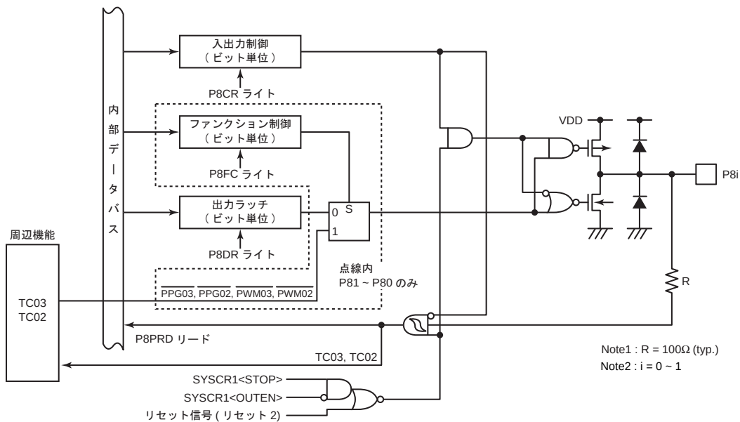
図 8-8 P8 ポート
