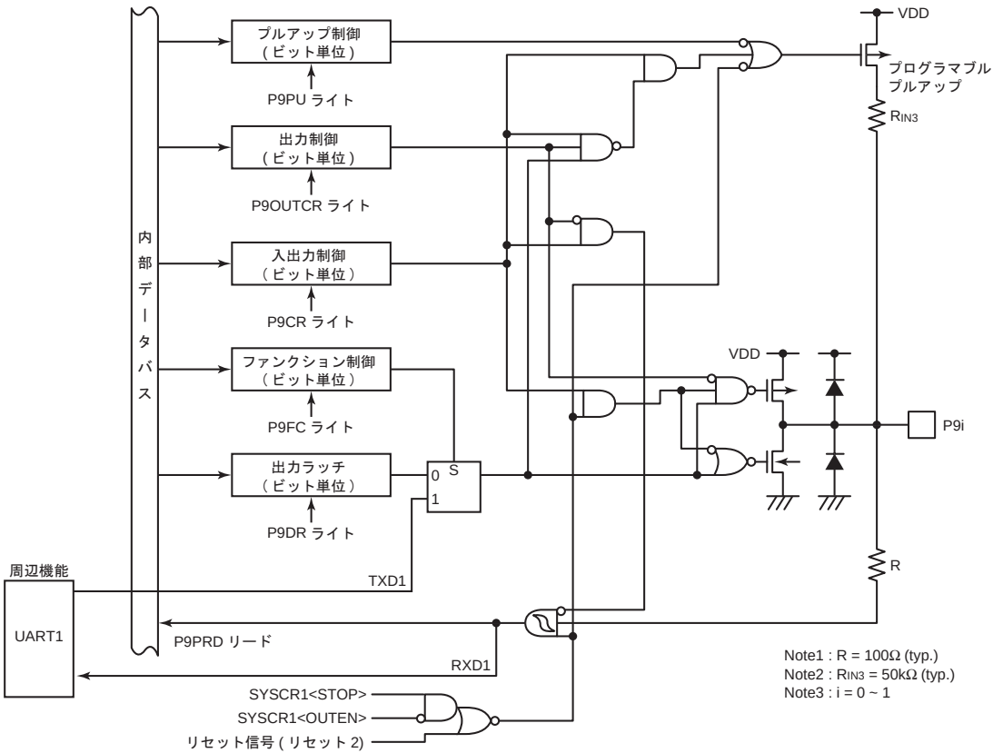
図 8-9 P9 ポート
