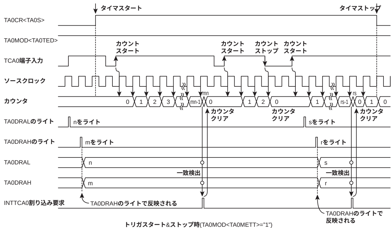
トリガスタート&ストップ時(TA0MOD<TA0METT>="1")
