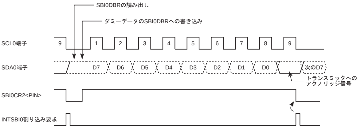
図 18-19 SBI0CR1<BC>=“000”，SBI0CR1<ACK>=“1” の場合
