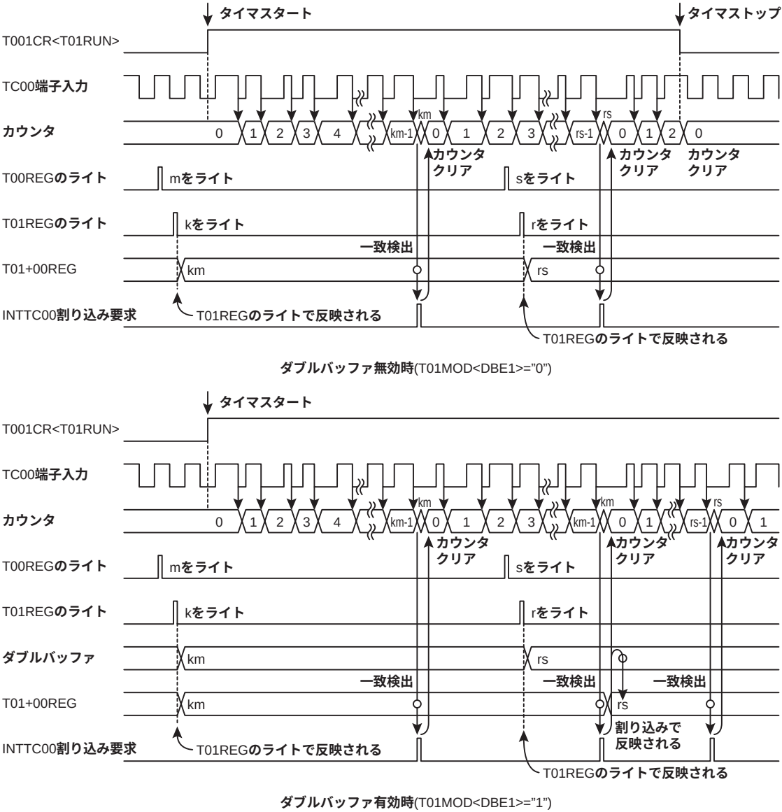
図 14-12 16 ビットイベントカウンタモードタイミングチャート
