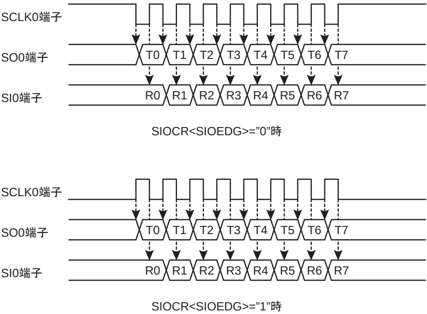
図 17-2 転送エッジ
