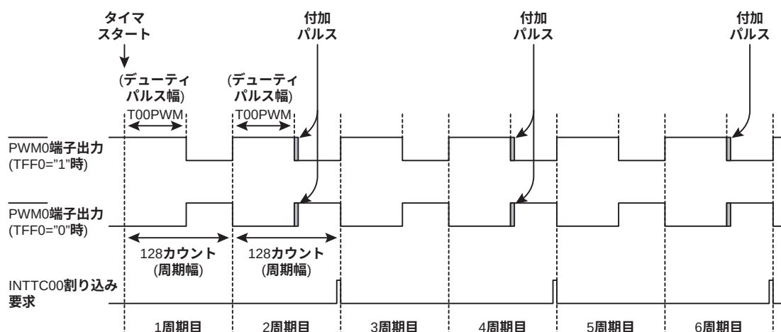
図 14-5 \overline{\text{PWM0}} パルス出力
