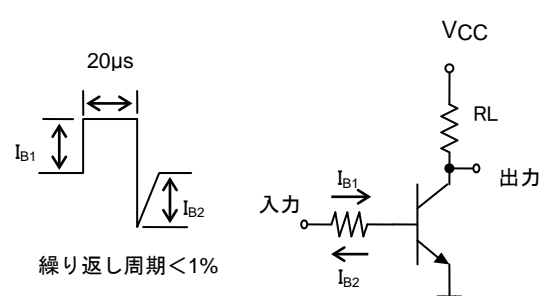
図 4. スイッチング時間測定回路
