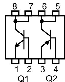
図1. 内部構造 (top view)
