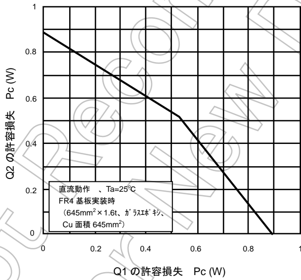
2 素子動作時の許容損失
