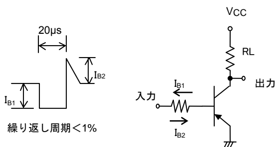
図 3. スイッチング時間測定回路
