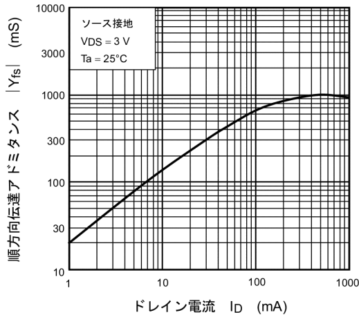
図 7.7 |Y_{fs}| - I_D
