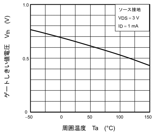
図 7.6 V_{th} - T_a
