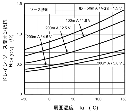
図 7.5 R_{DS(ON)} - T_a
