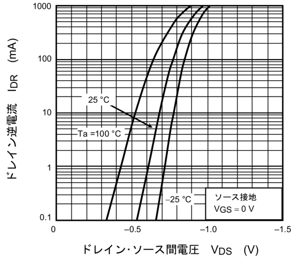
図 7.8 I_{DR} - V_{DS}
