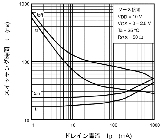
図 7.10 t - I_D
