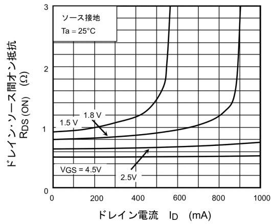
図 7.4 R_{DS(ON)} - I_D
