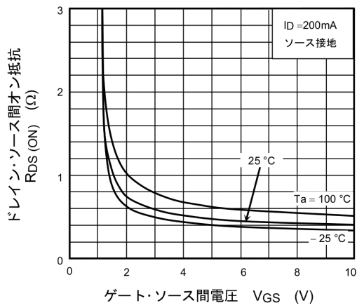
図 7.3 R_{DS(ON)} - V_{GS}
