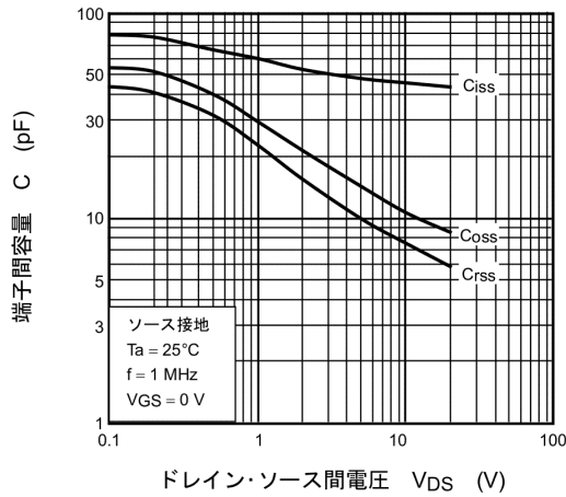
図 7.9 C - V_{DS}
