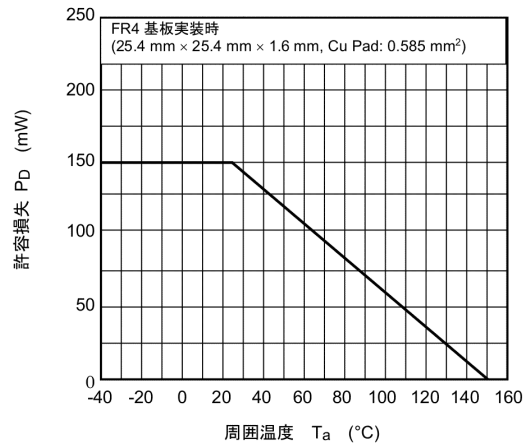
図 7.12 P_D - T_a
