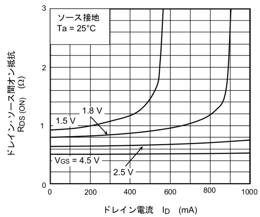
図 7.4 R_{DS(ON)} - I_D
