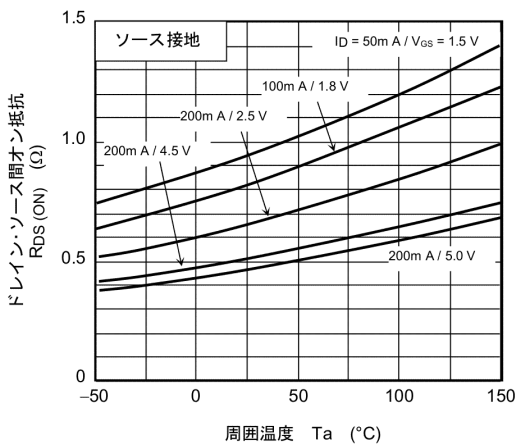
図 7.5 R_{DS(ON)} - T_a
