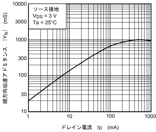
図 7.7 |Y_{fs}| - I_D
