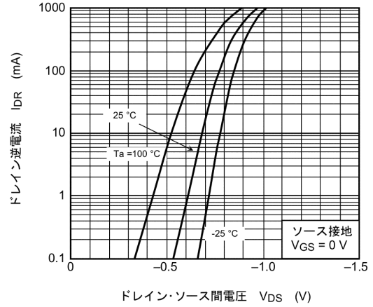
図 7.8 I_{DR} - V_{DS}
