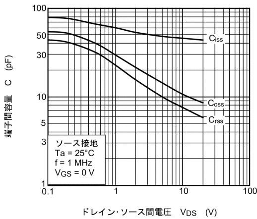
図 7.9 C - V_{DS}
