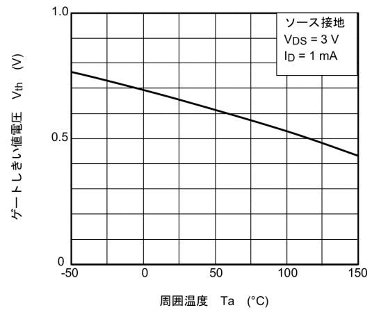
図 7.6 V_{th} - T_a
