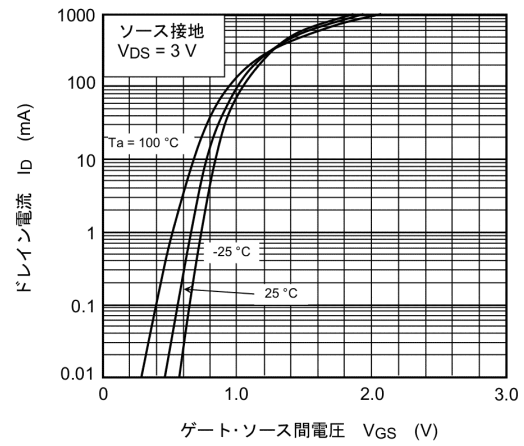
図 7.2 I_D - V_{GS}
