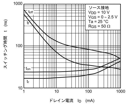
図 7.10 t - I_D
