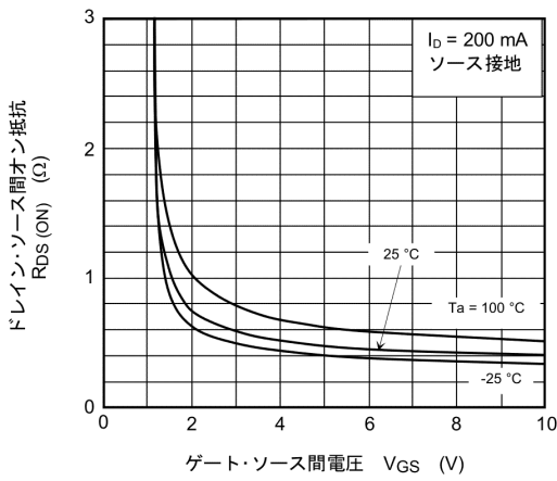
図 7.3 R_{DS(ON)} - V_{GS}
