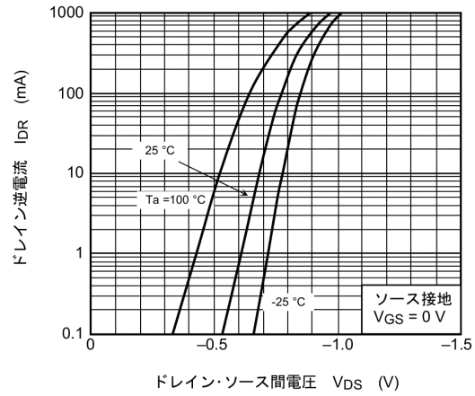
図 7.8 I_{DR} - V_{DS}
