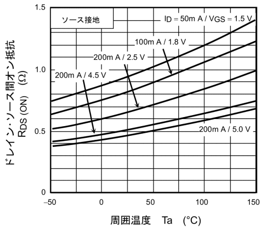
図 7.5 R_{DS(ON)} - T_a
