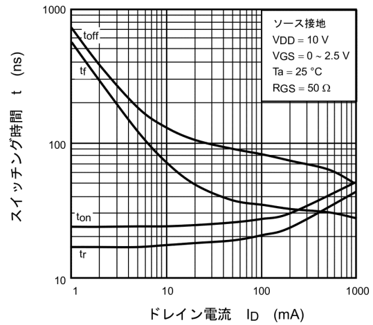
図 7.10 t - I_D
