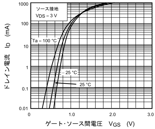
図 7.2 I_D - V_{GS}
