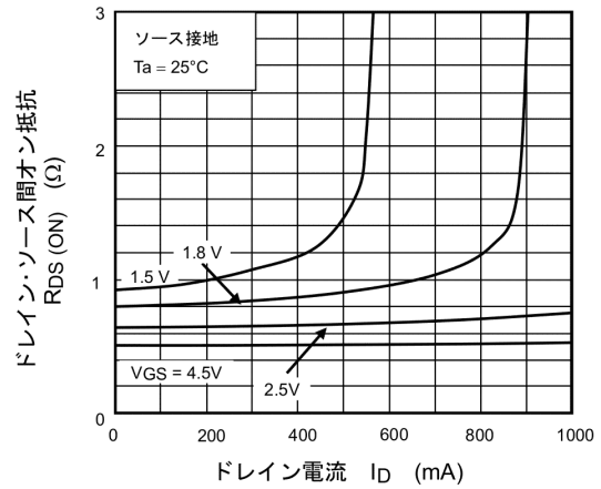
図 7.4 R_{DS(ON)} - I_D
