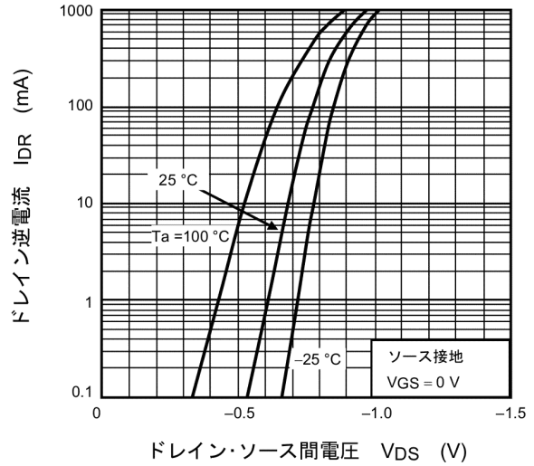
図 7.8 I_{DR} - V_{DS}
