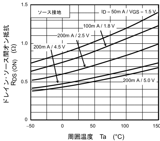
図 7.5 R_{DS(ON)} - T_a
