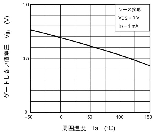
図 7.6 V_{th} - T_a
