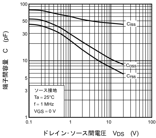
図 7.9 C - V_{DS}
