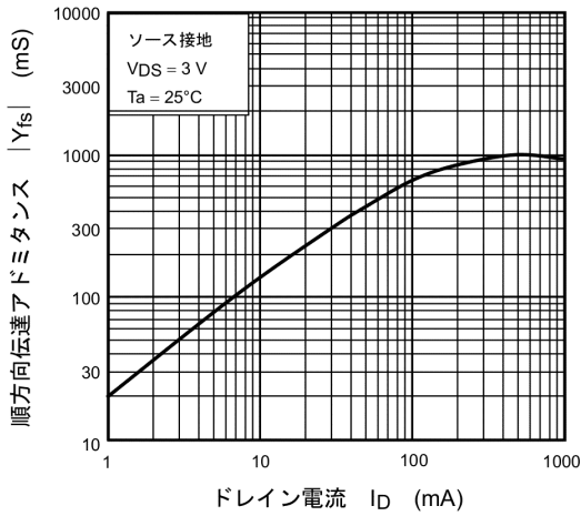
図 7.7 |Y_{fs}| - I_D
