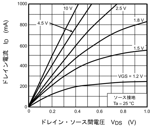
図 7.1 I_D - V_{DS}
