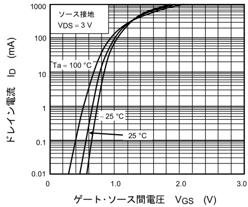
図 7.2 I_D - V_{GS}
