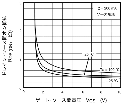
図 7.3 R_{DS(ON)} - V_{GS}
