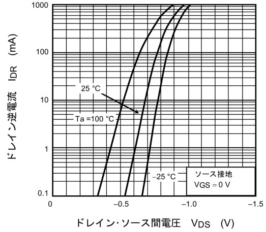
図 7.8 I_{DR} - V_{DS}
