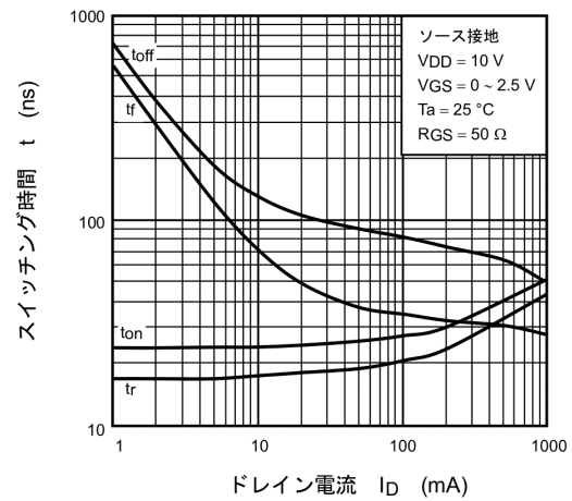
図 7.10 t - I_D
