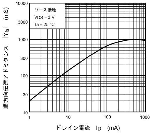
図 7.7 |Y_{fs}| - I_D
