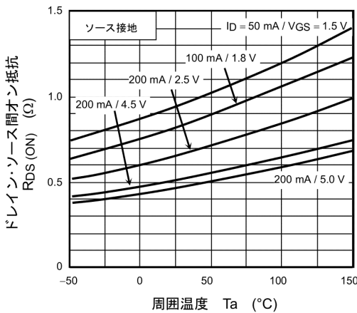
図 7.5 R_{DS(ON)} - T_a
