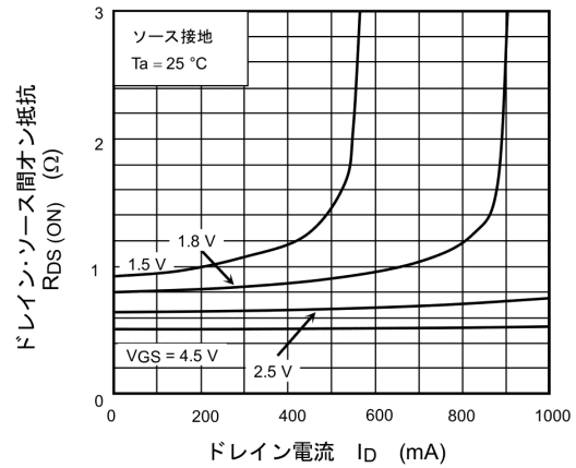
図 7.4 R_{DS(ON)} - I_D
