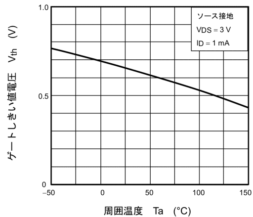
図 7.6 V_{th} - T_a
