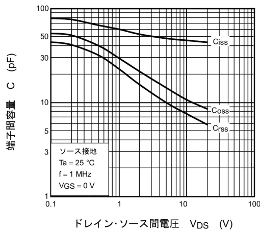
図 7.9 C - V_{DS}
