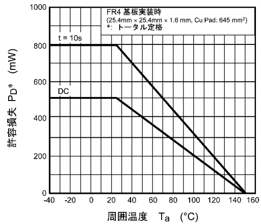
図 7.12 P_D - T_a
