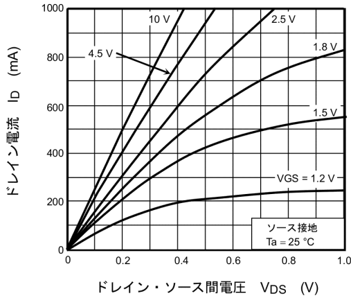
図 7.1 I_D - V_{DS}
