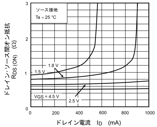
図 7.4 R_{DS(ON)} - I_D
