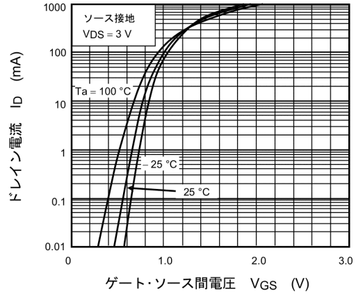
図 7.2 I_D - V_{GS}
