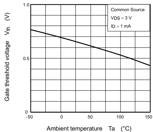
Fig. 7.6 V_{th} - T_a
