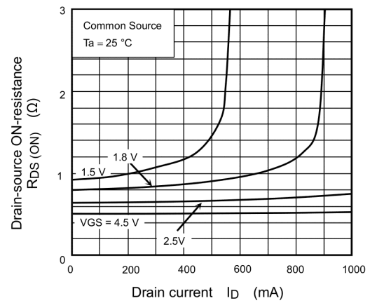
Fig. 7.4 R_{DS(ON)} - I_D
