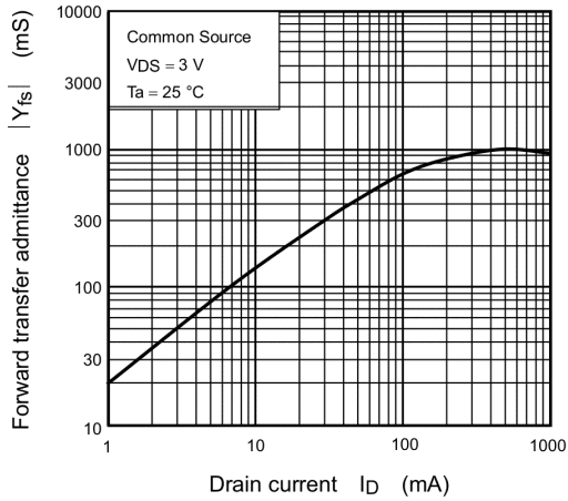
Fig. 7.7 |Y_{fs}| - I_D
