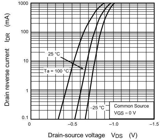
Fig. 7.8 I_{DR} - V_{DS}
