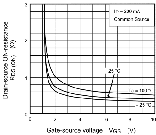
Fig. 7.3 R_{DS(ON)} - V_{GS}
