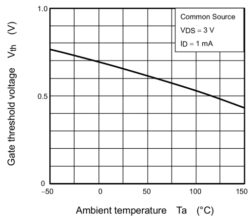
Fig. 7.6 V_{th} - T_a
