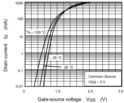
Fig. 7.2 I_D - V_{GS}
