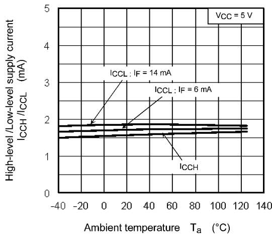
Fig. 12.2.5 I_{CH} / I_{CLL} - T_a
