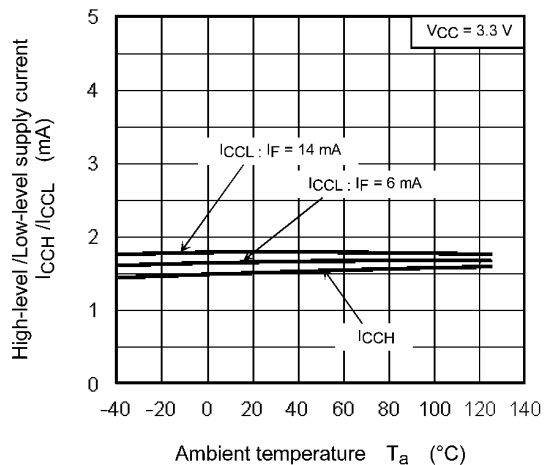
Fig. 12.2.6 I_{CH} / I_{CLL} - T_a
