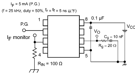
図 13.1.5 I CCH 測定回路
