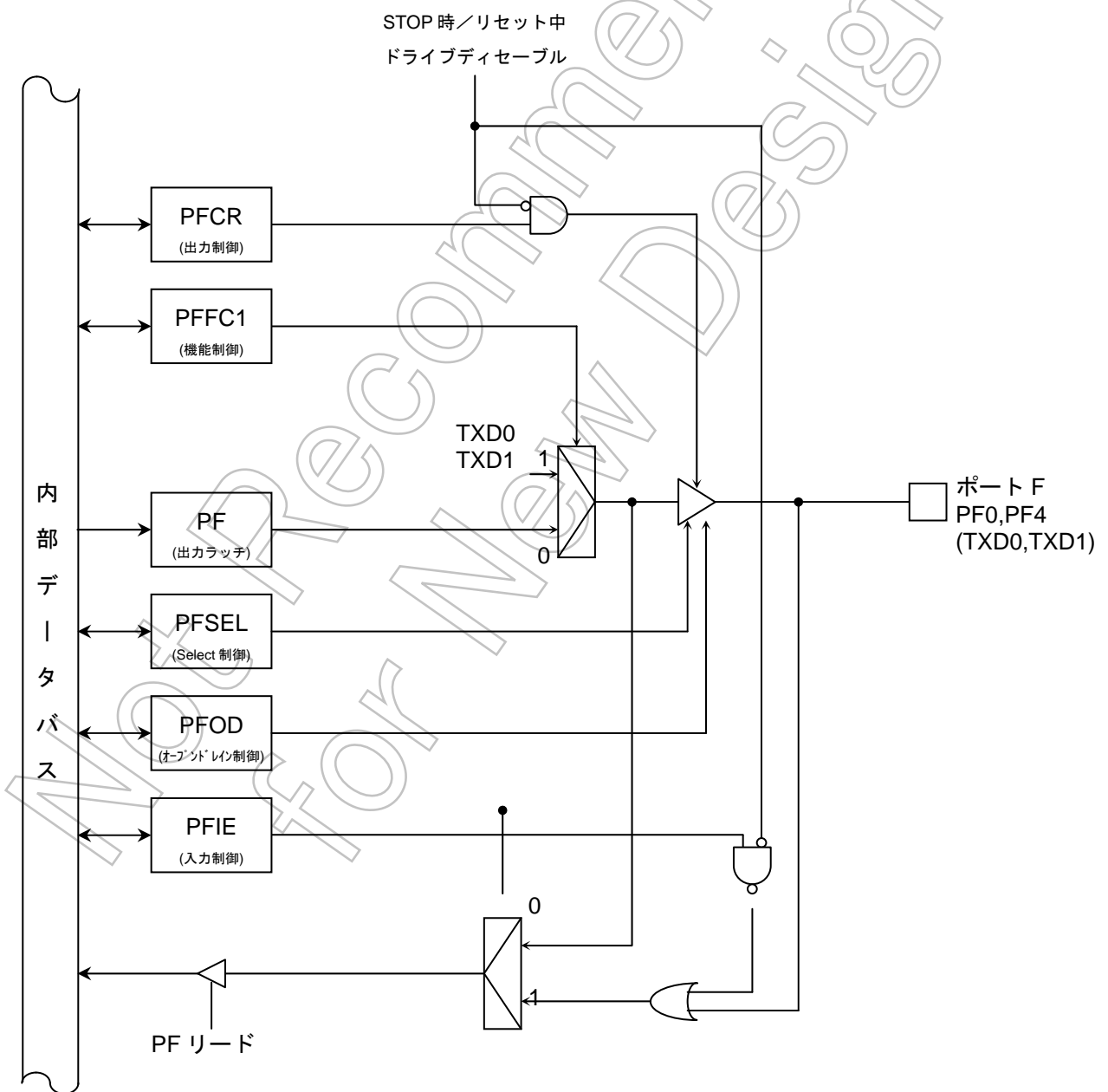
図 7-24 ポート F(PF0,PF4)
