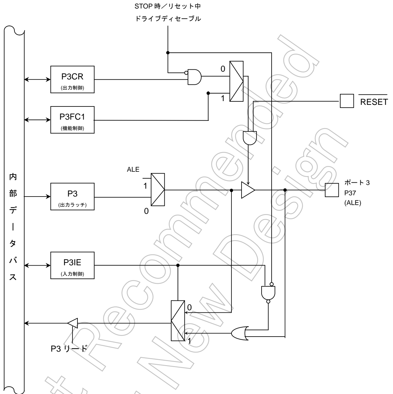
図 7-7 ポート 3 (P37)
