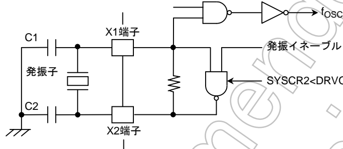
図 5.5.1 発振器のドライブ能力
