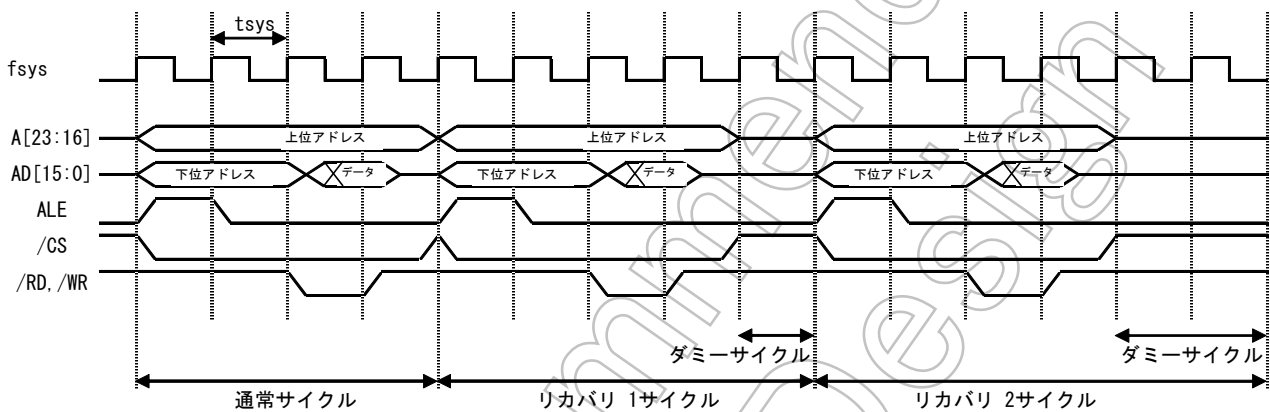
図 8.4.7 リカバリタイム挿入時のタイミング
