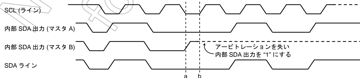
図 14.5.10.1 アービトレイションロスト
