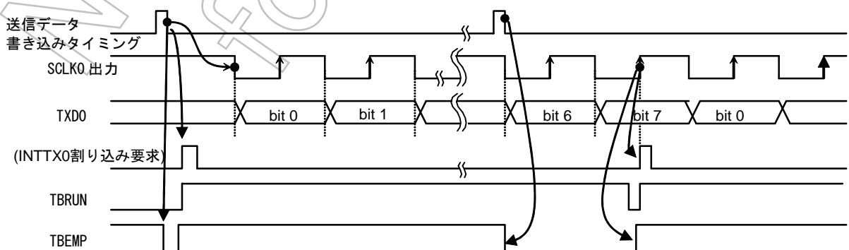
\langle WBUF \rangle = "1" (ダブルバッファ許可) の場合 (バッファ 2 にデータがある場合)
