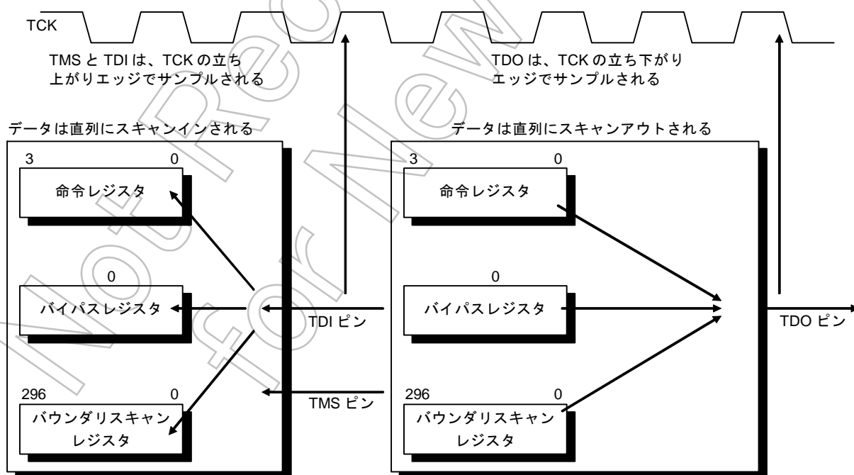
図 20.6 JTAG テストアクセスポート
