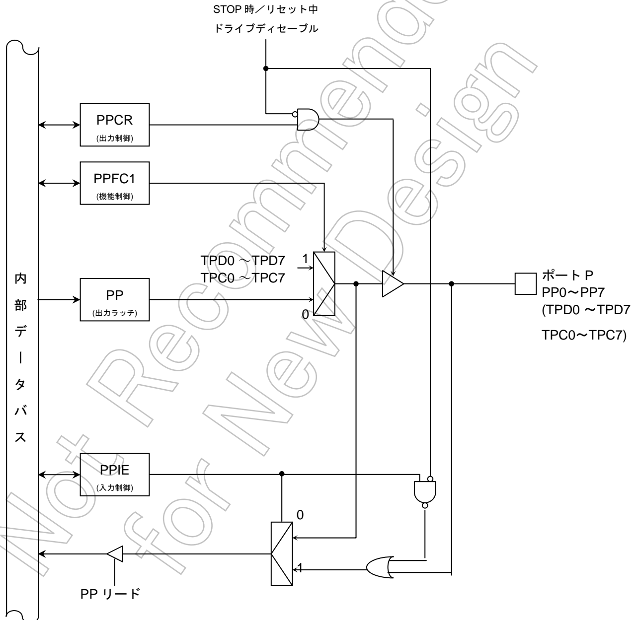
図 7-56 ポート P
