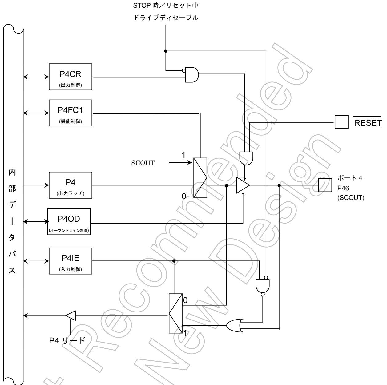
図 7-9 ポート 4 (P46)
