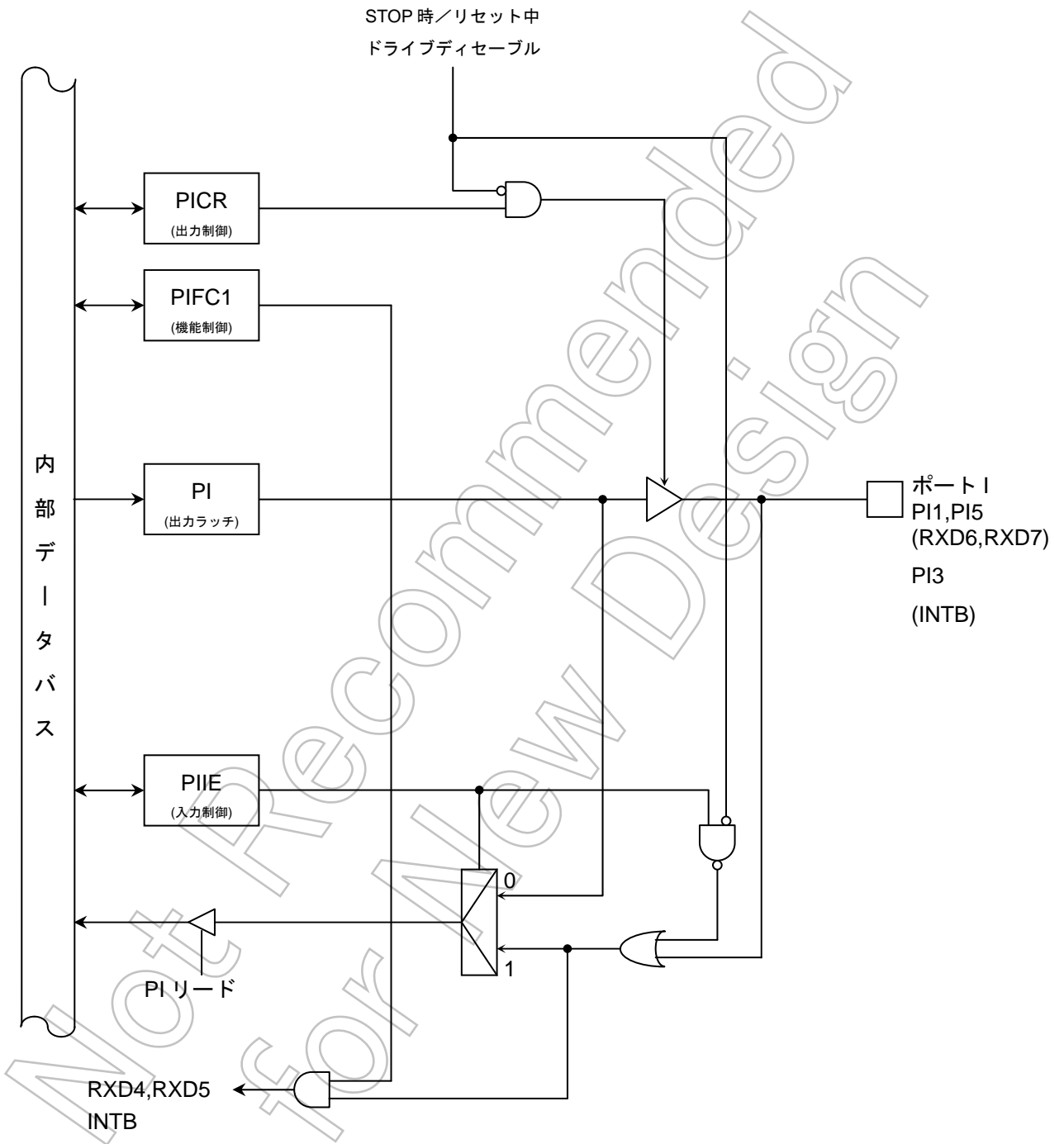
図 7-36 ポート I (PI1, PI5, PI3)
