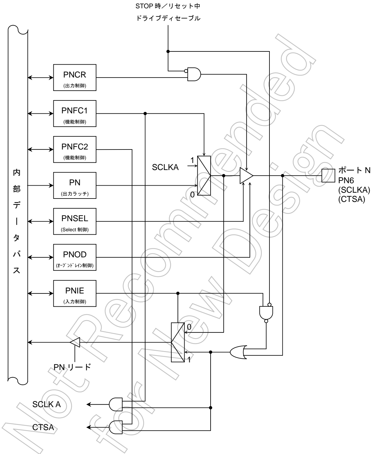
図 7-54 ポート N(PN6)
