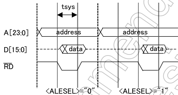
図 8. 3. 8 SYSCR3&lt;ALESEL&gt;設定値と外部バスオペレーション
