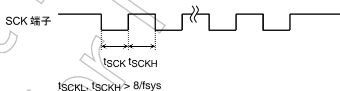
図 14.7.1.4 外部クロック入力時の最大転送周波数
