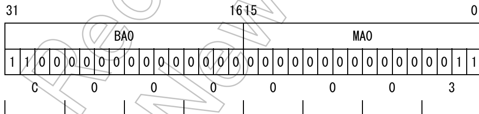
ベース/マスクアドレスレジスタ (BMA0) 設定値
