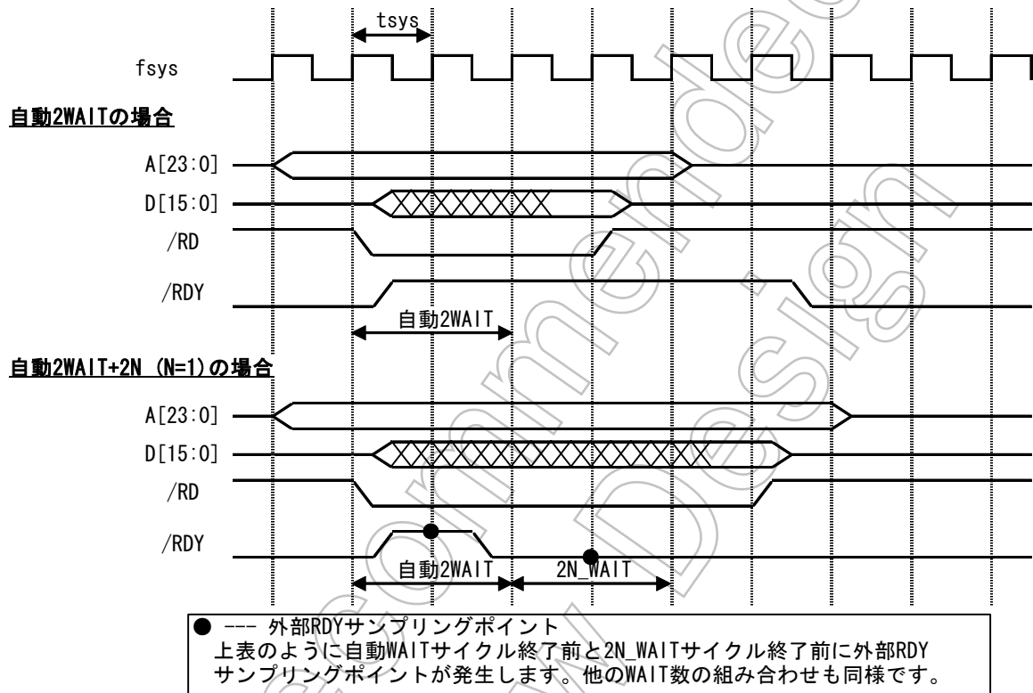
図 8.3.7 RDY 入力とウェイトオペレーションタイミング図
