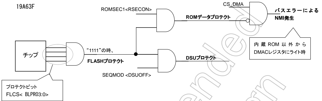
図 22.1 各種プロテクト状態概略
