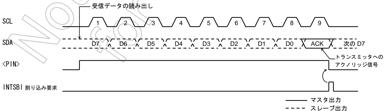
図 14.6.3.2 <BC2:0> = “000”, <ACK> = “1” の場合 (レシーバモード)
