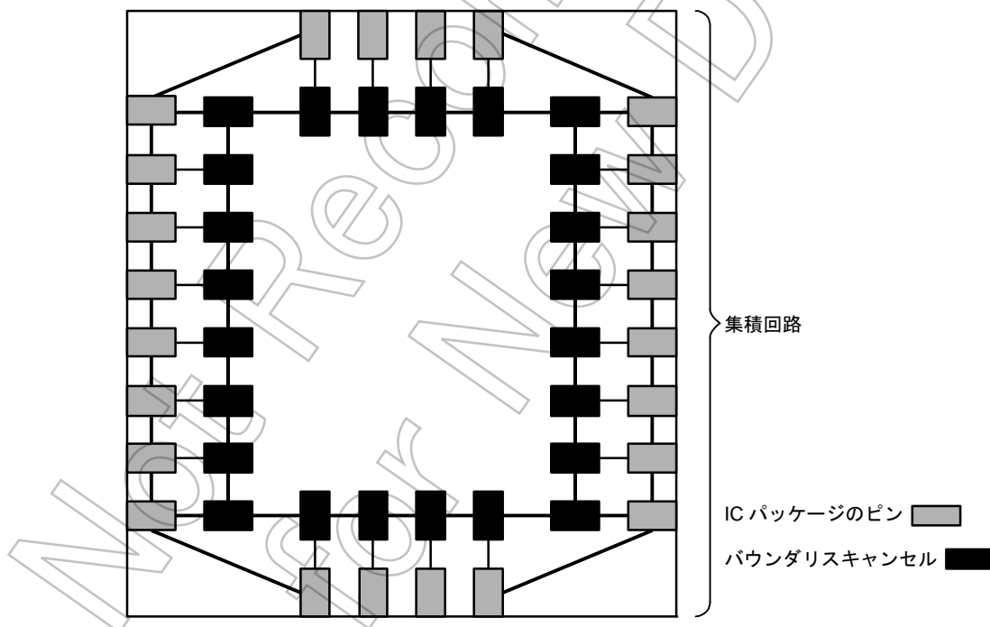
図 20.1 JTAG バウンダリスキャンセル
