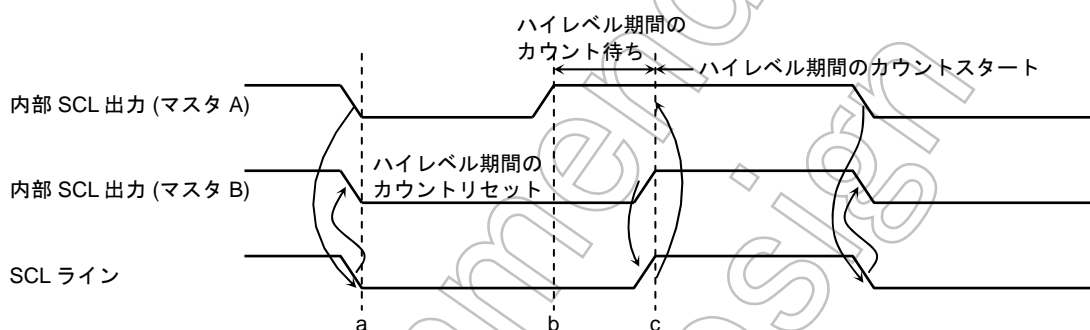
図 14.5.3.2 クロック同期化の例
