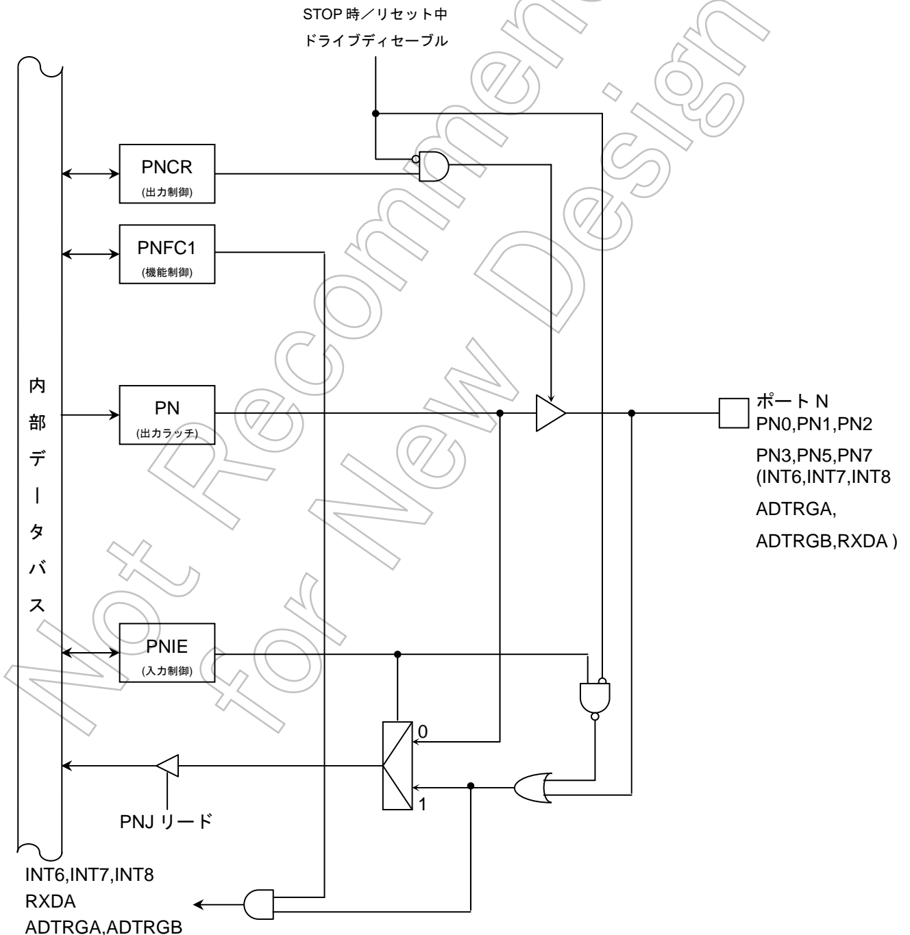
図 7-52 ポート N (PN0,PN1,PN2,PN3,PN5,PN7)
