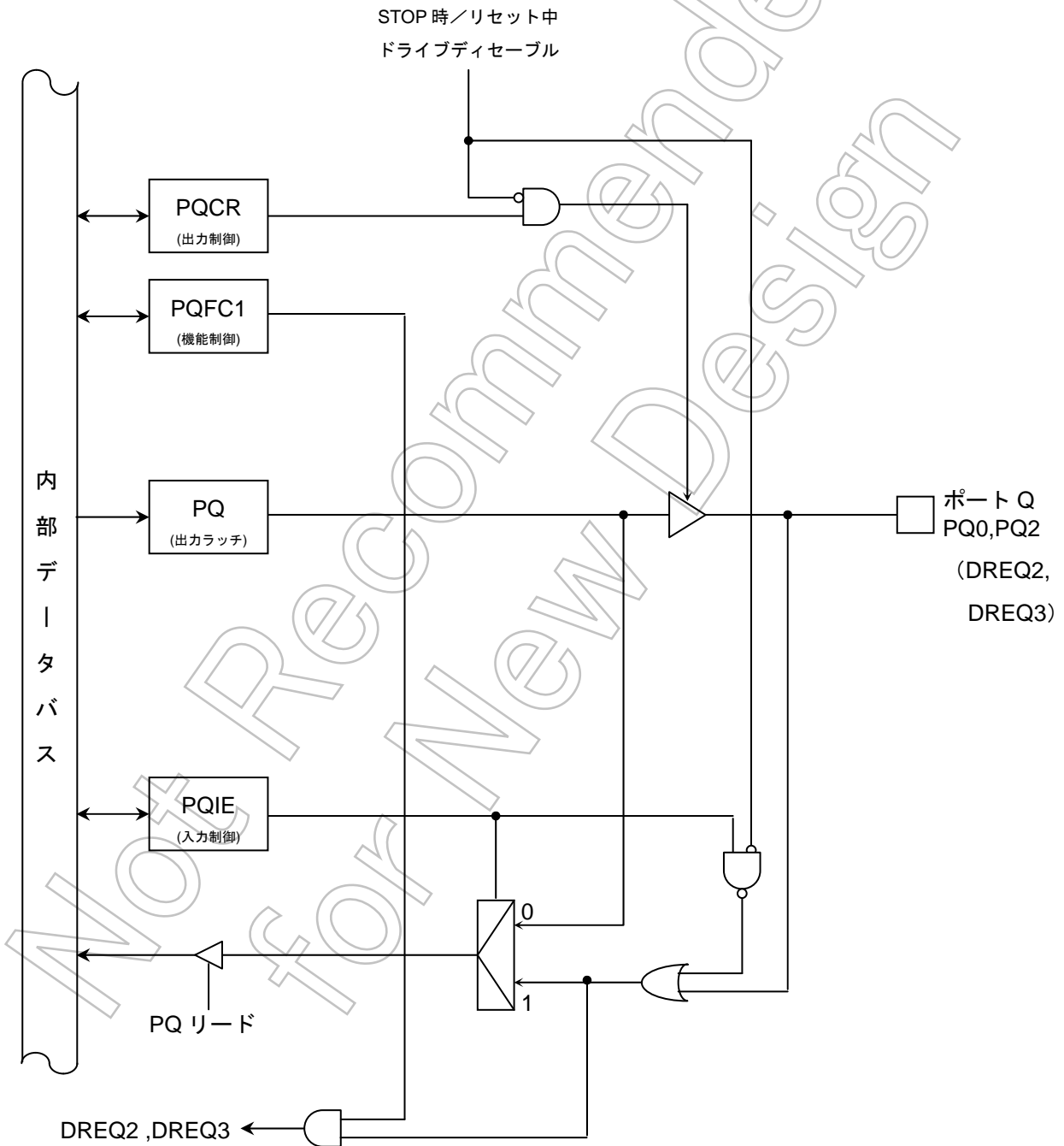
図 7-57 ポート Q(PQ0,PQ2)
