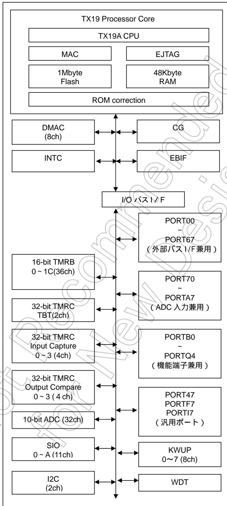
図 1.1 TMP19A63F10XBG ブロック図
