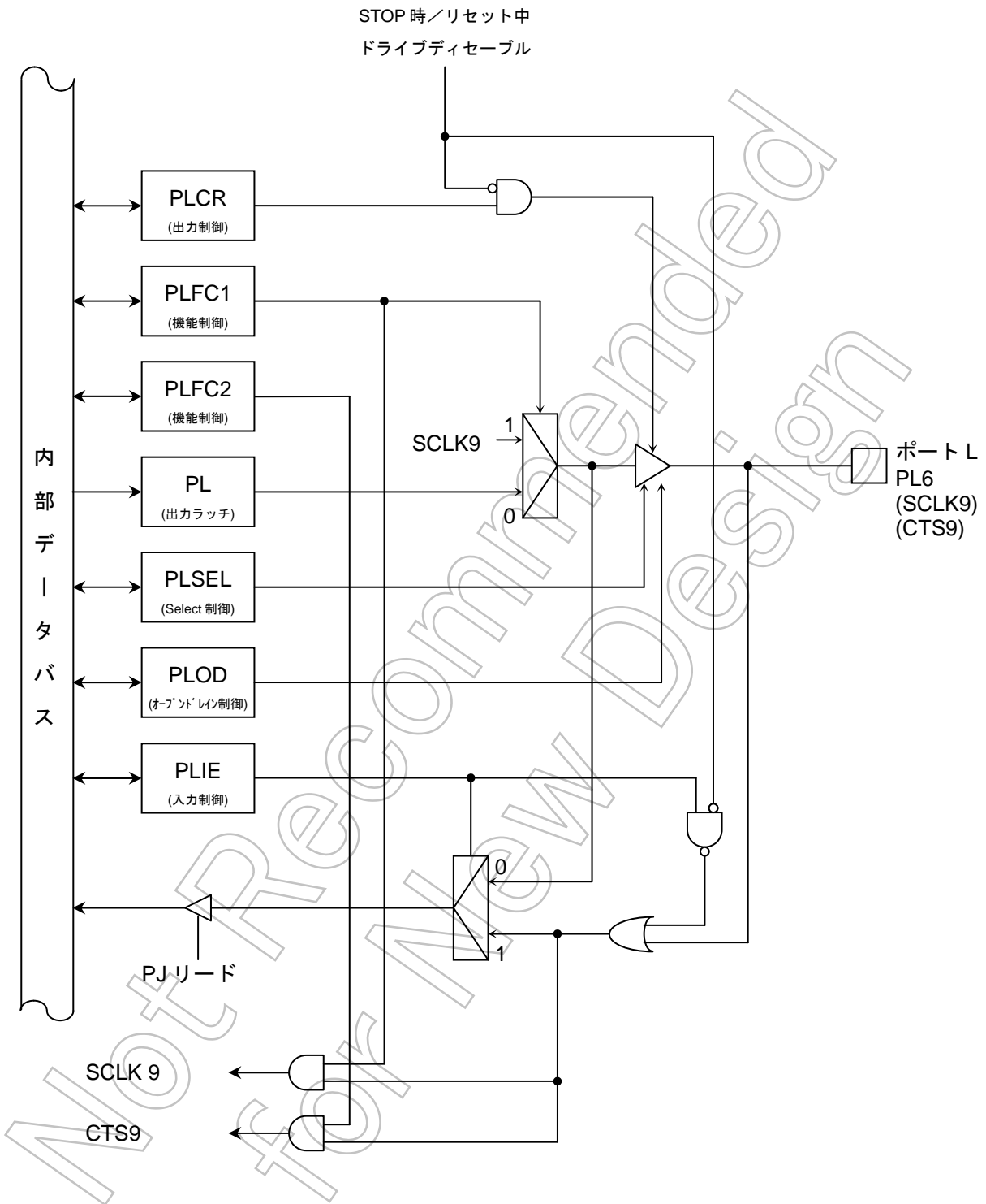
図 7-49 ポート L(PL6)
