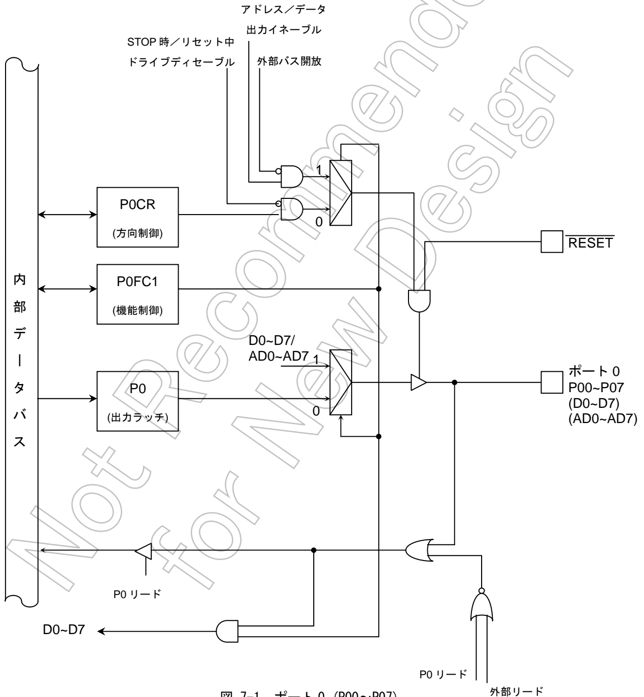
図 7-1 ポート 0 (P00~P07)
