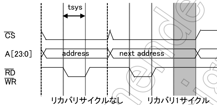
図 8.3.10 CS リカバリタイム挿入時のタイミング
