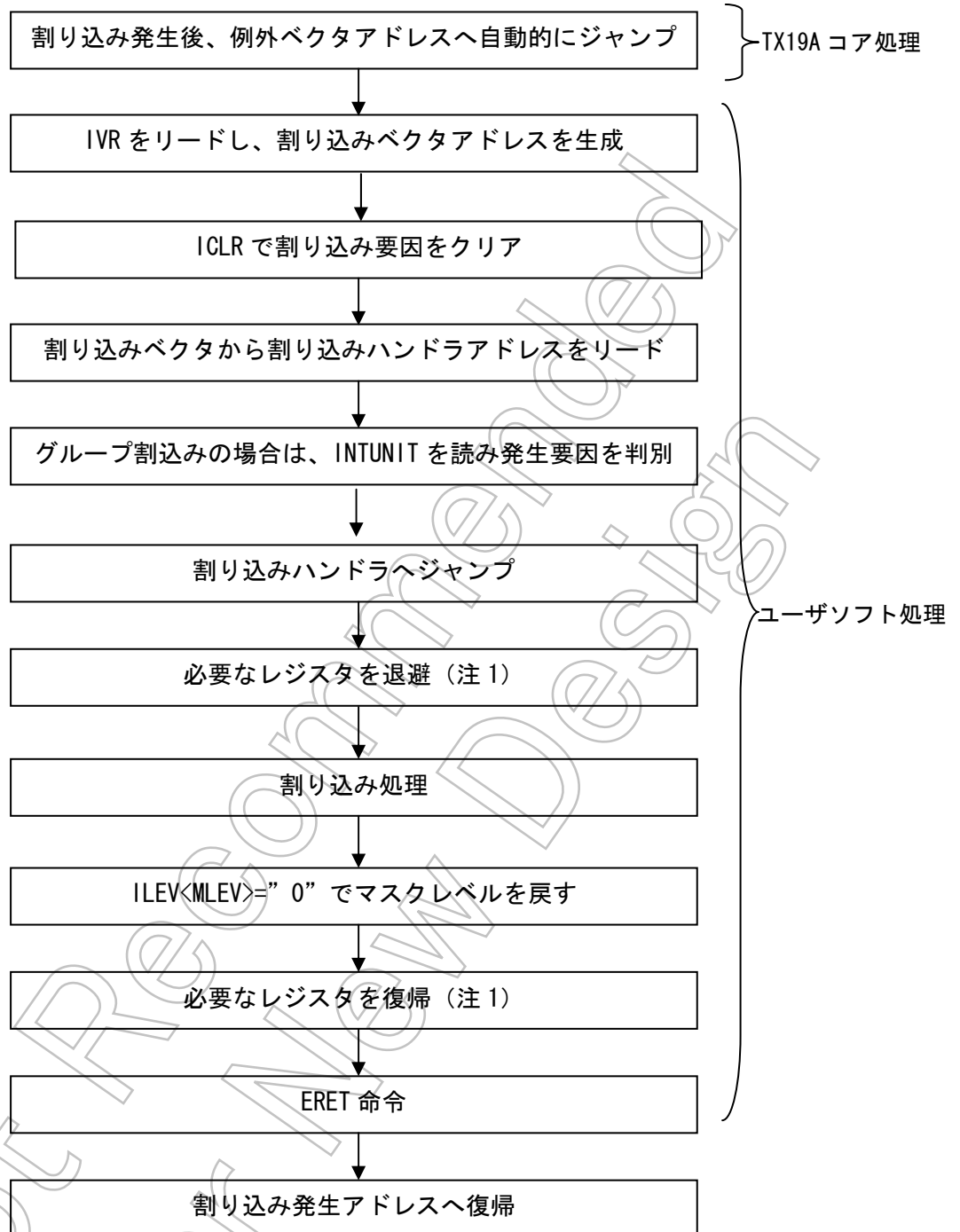
図 6.8.5 ハードウェア割り込みの基本動作例
