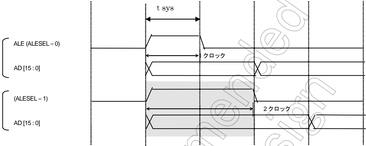
図 8.4.5 ALE のアサート時間
