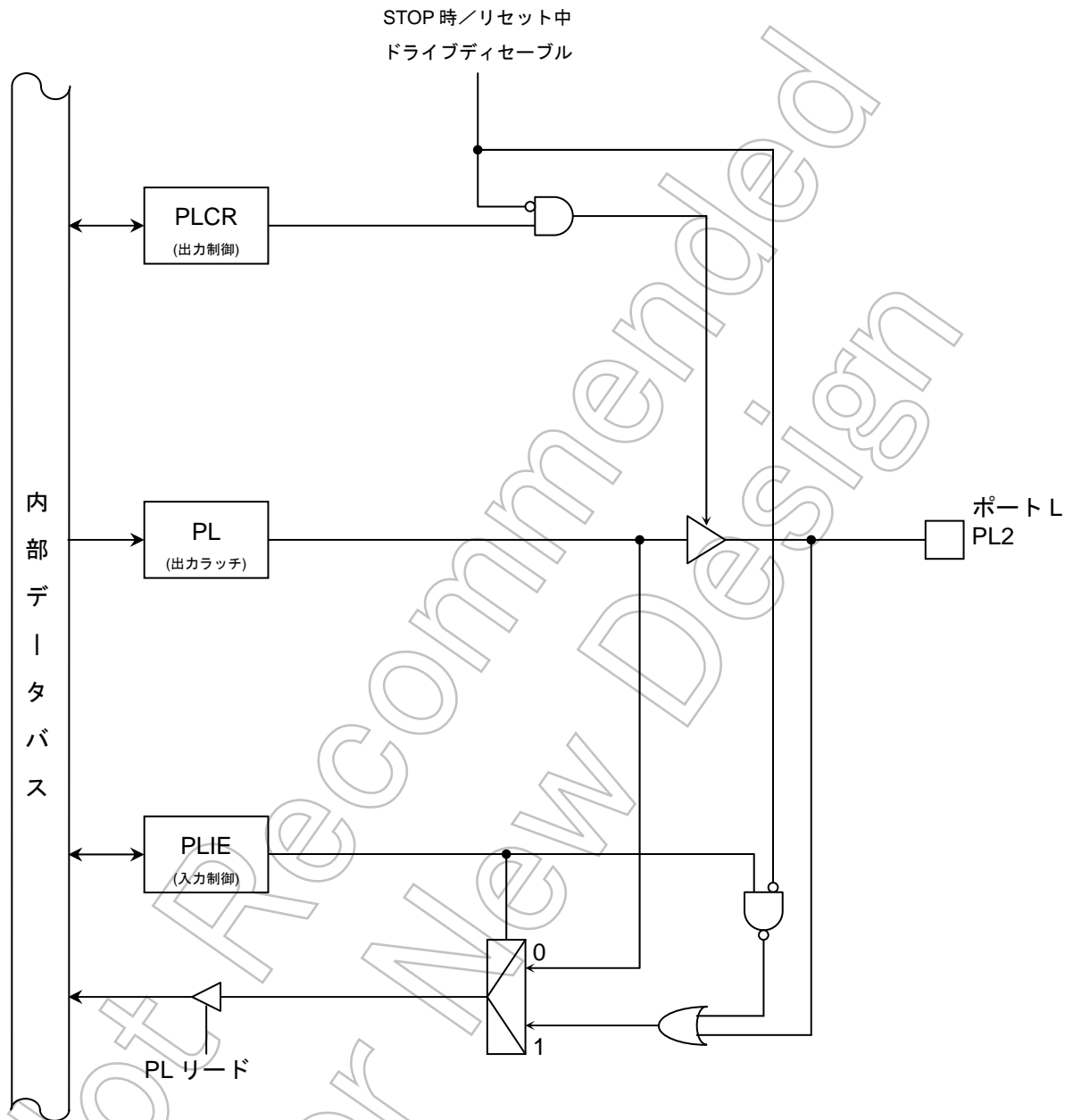
図 7-46 ポート L(PL2)
