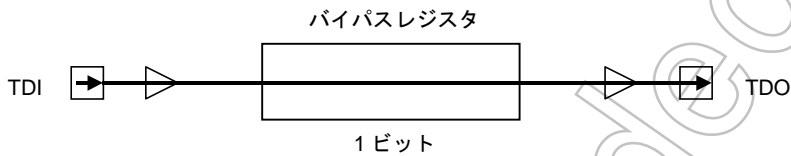
図 20.11 バイパスレジスタが選択されているときのテストデータの流れ
