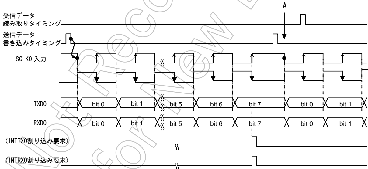
<WBUF>= “0” （ダブルバッファ不許可）の場合
