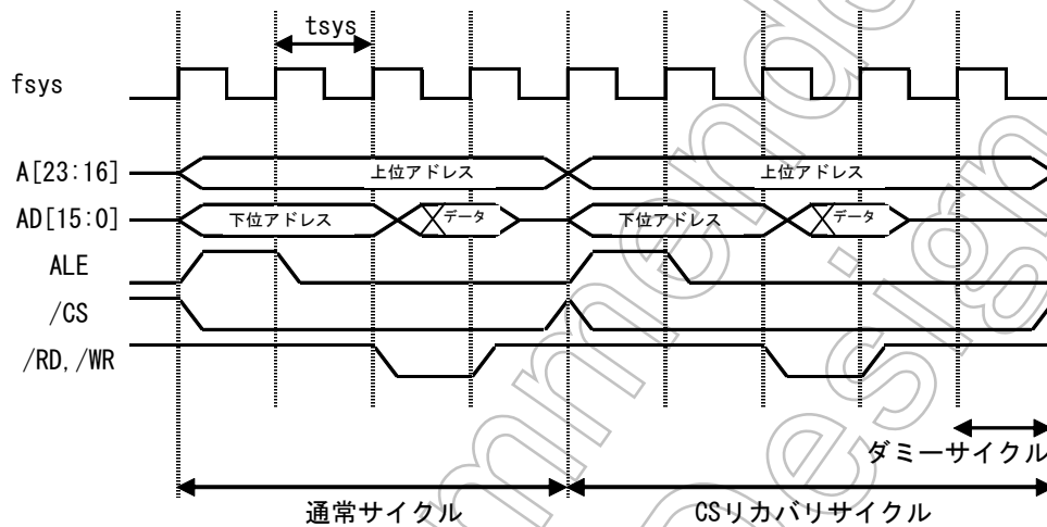
図 8.4.8 CSリカバリタイム挿入時
