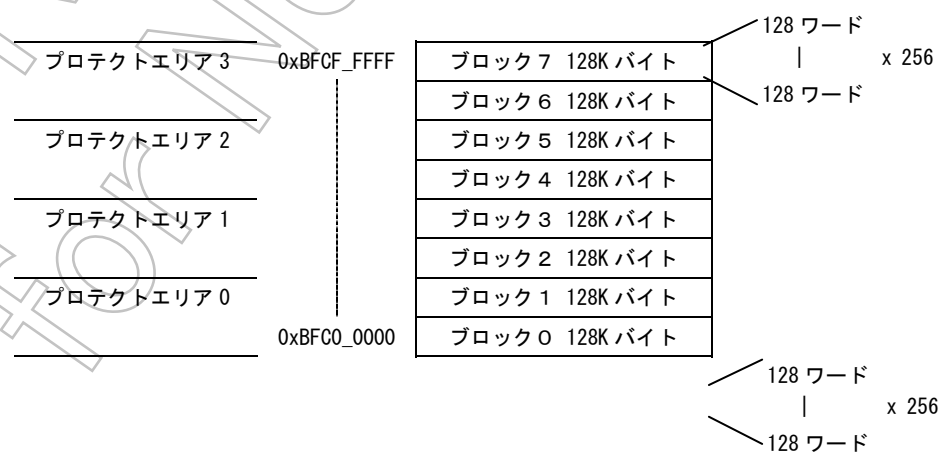
図 21.10 フラッシュメモリのブロック構成
