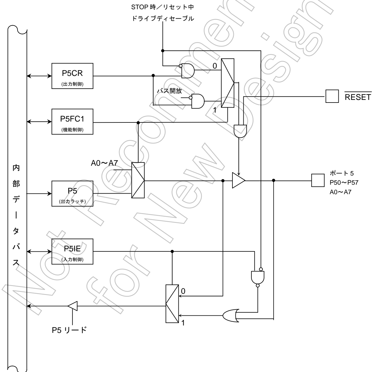
図 7-11 ポート 5 (P50~P57)
