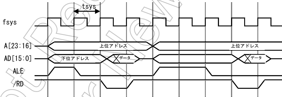
図 8.4.6 リードオペレーションタイミング図 (ALE 1クロックおよび2クロック)
