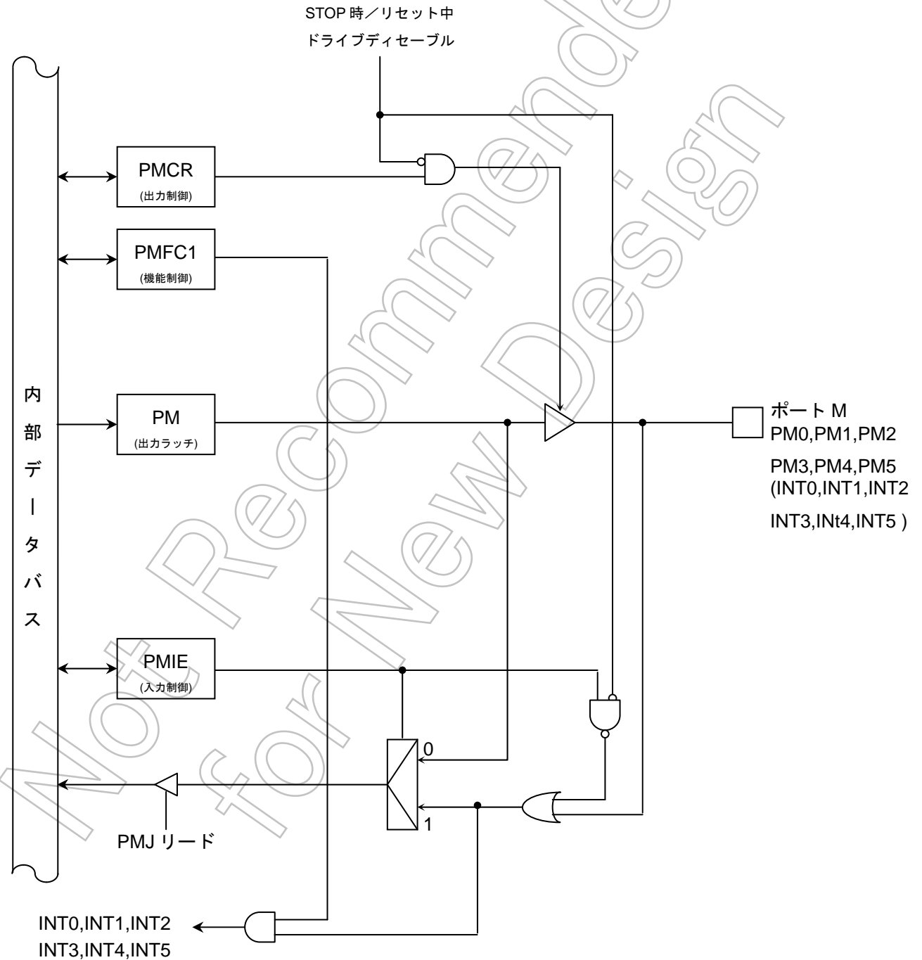
図 7-50 ポート M(PM0,PM1,PM2,PM3,PM4,PM5)
