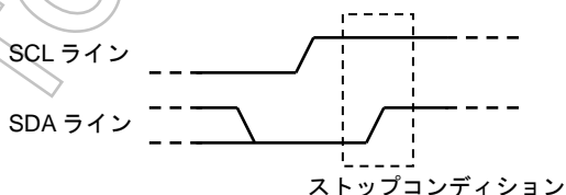
図 14.5.7.2 ストップコンディションの発生
