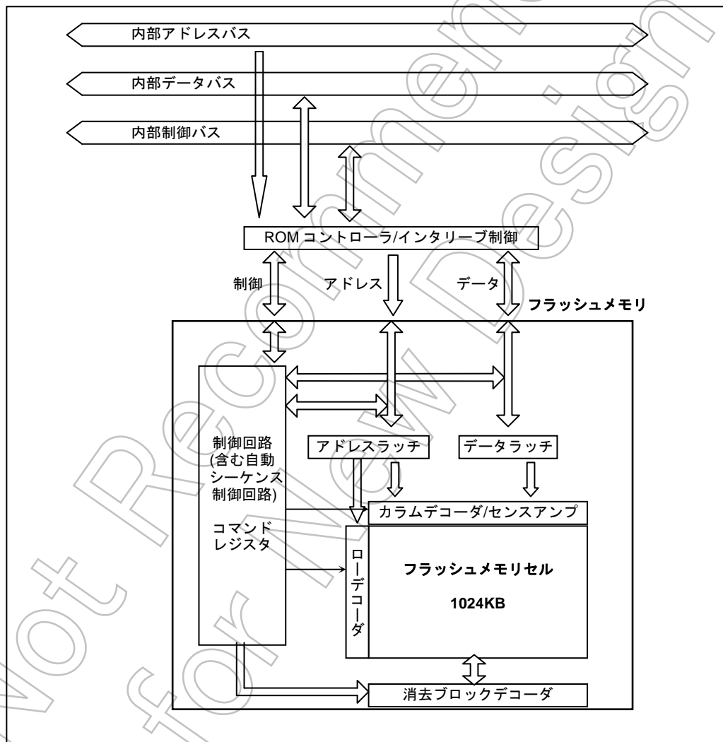
図 21.1 フラッシュ部ブロック図
