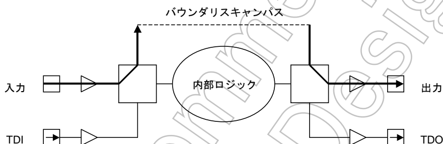
図 20.8 EXTEST 命令が選択されているときのテストデータの流れ
