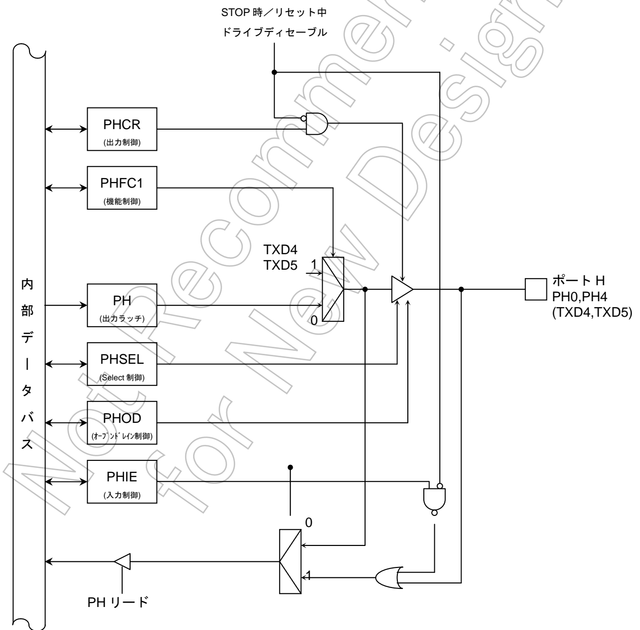
図 7-32 ポート H(PH0,PH4)
