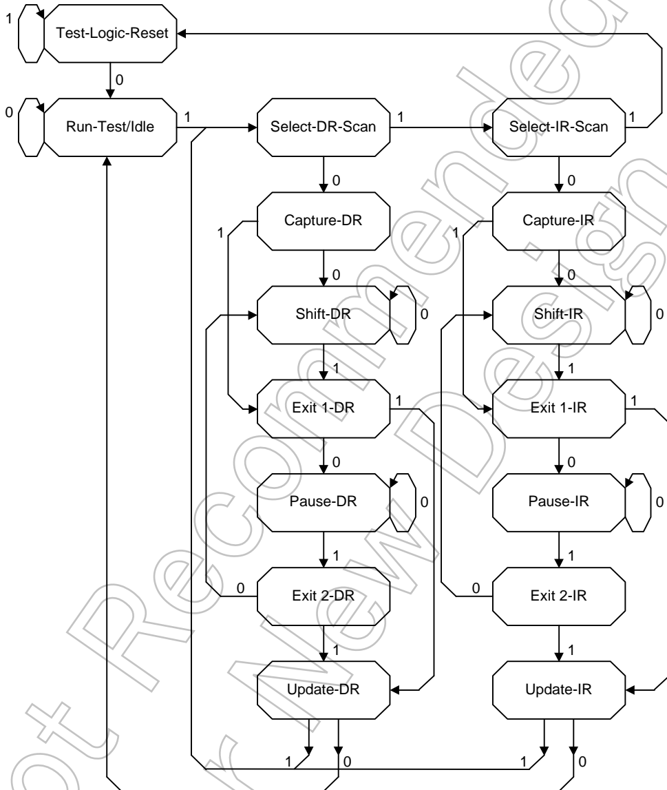
図 20.7 TAP コントローラの状態遷移図
