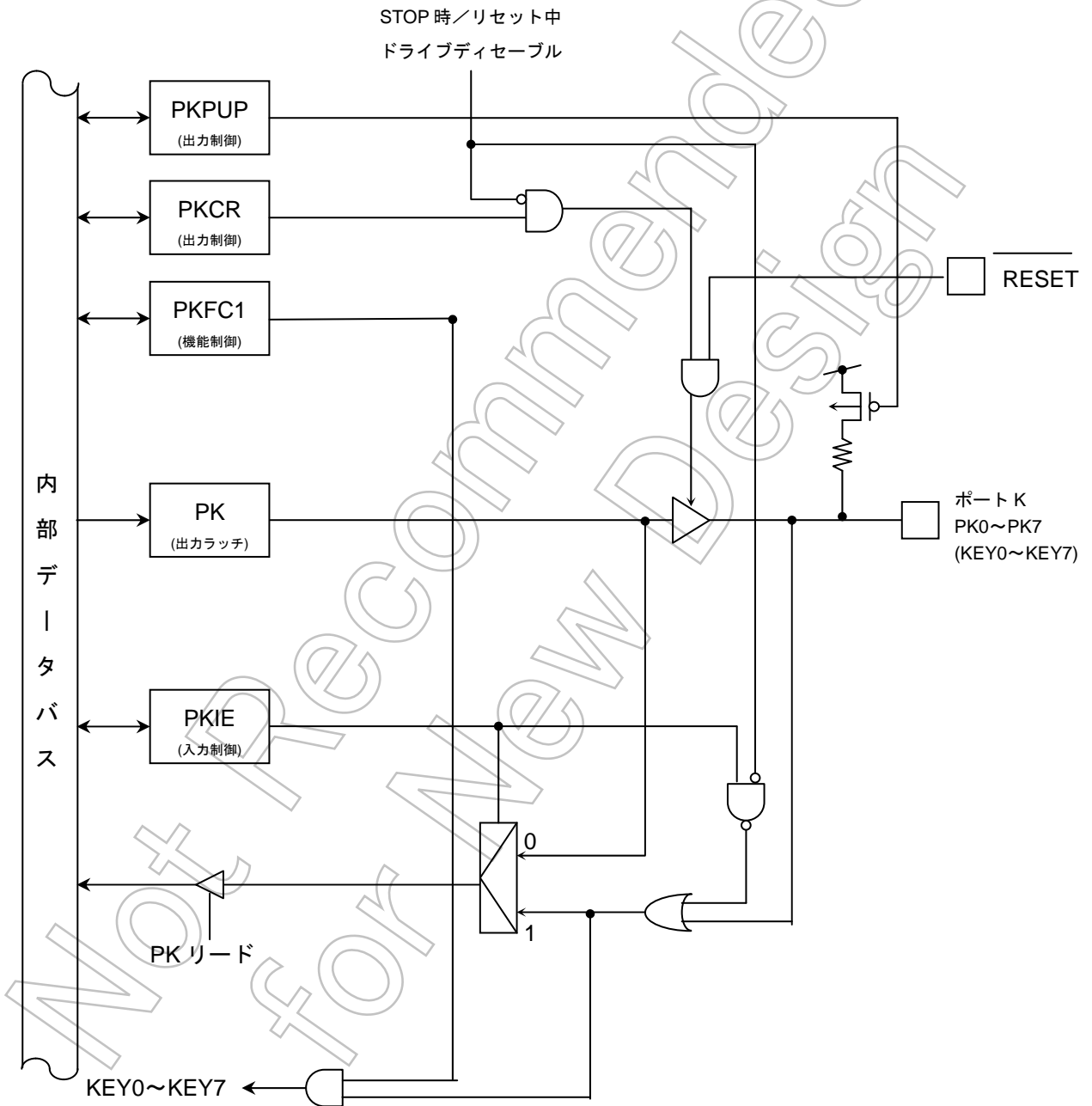
図 7-44 ポート K (PK0~PK7)
