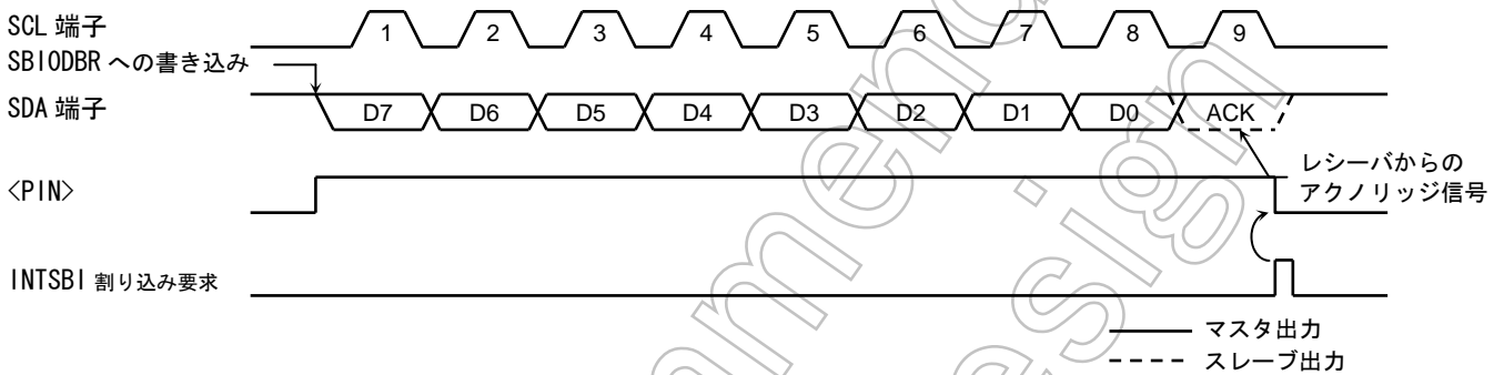
図 14.6.3.1 <BC2:0> = “000”, <ACK> = “1” の場合 (トランスミッタモード)
