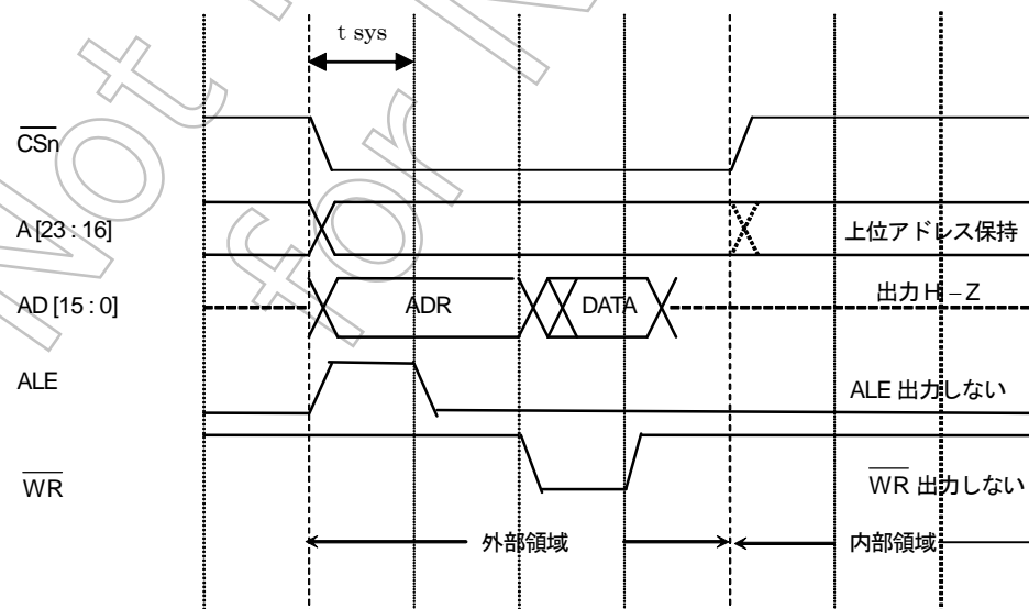
図 8.4.2 ライトオペレーションタイミング図
