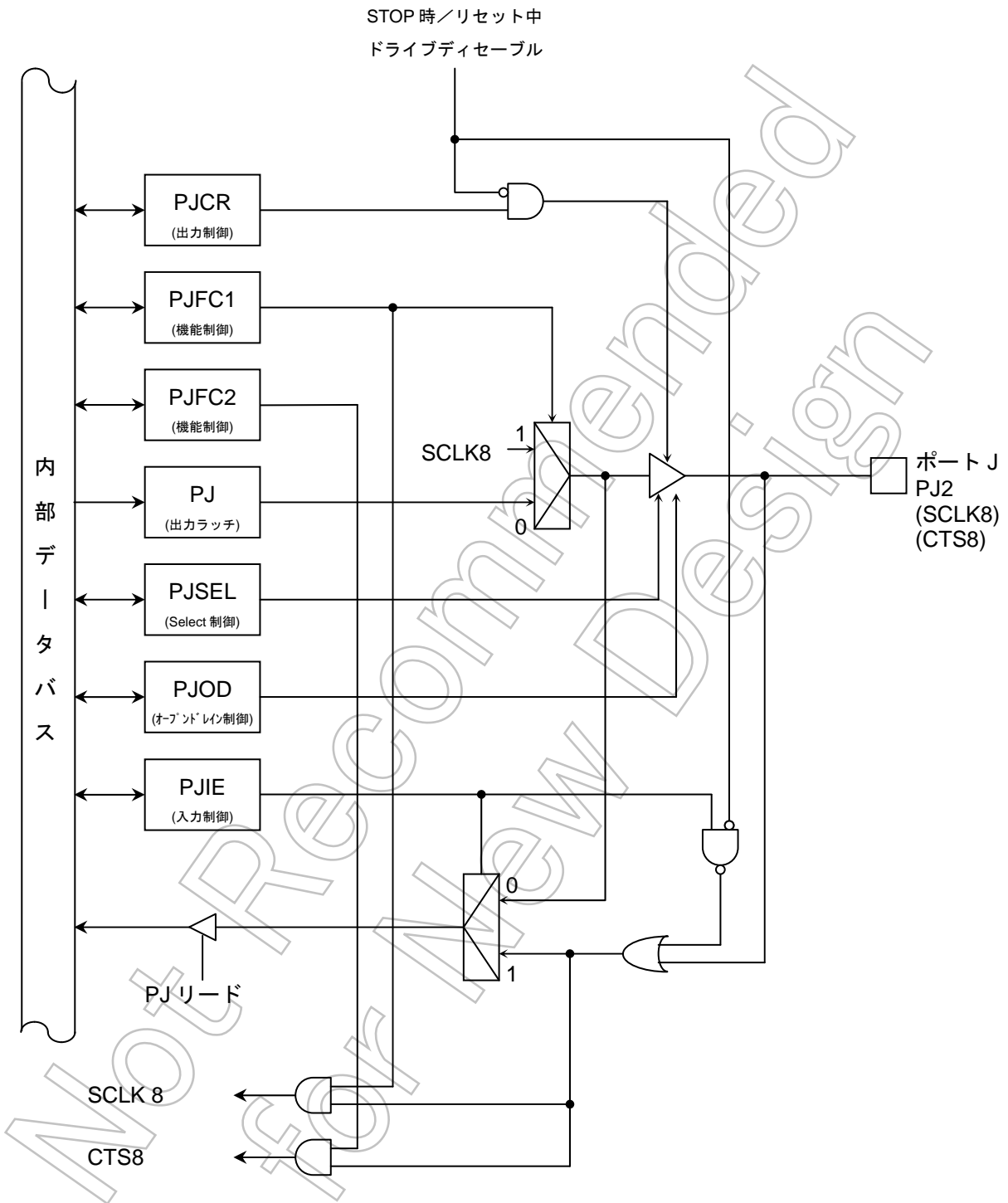
図 7-41 ポート J(PJ2)
