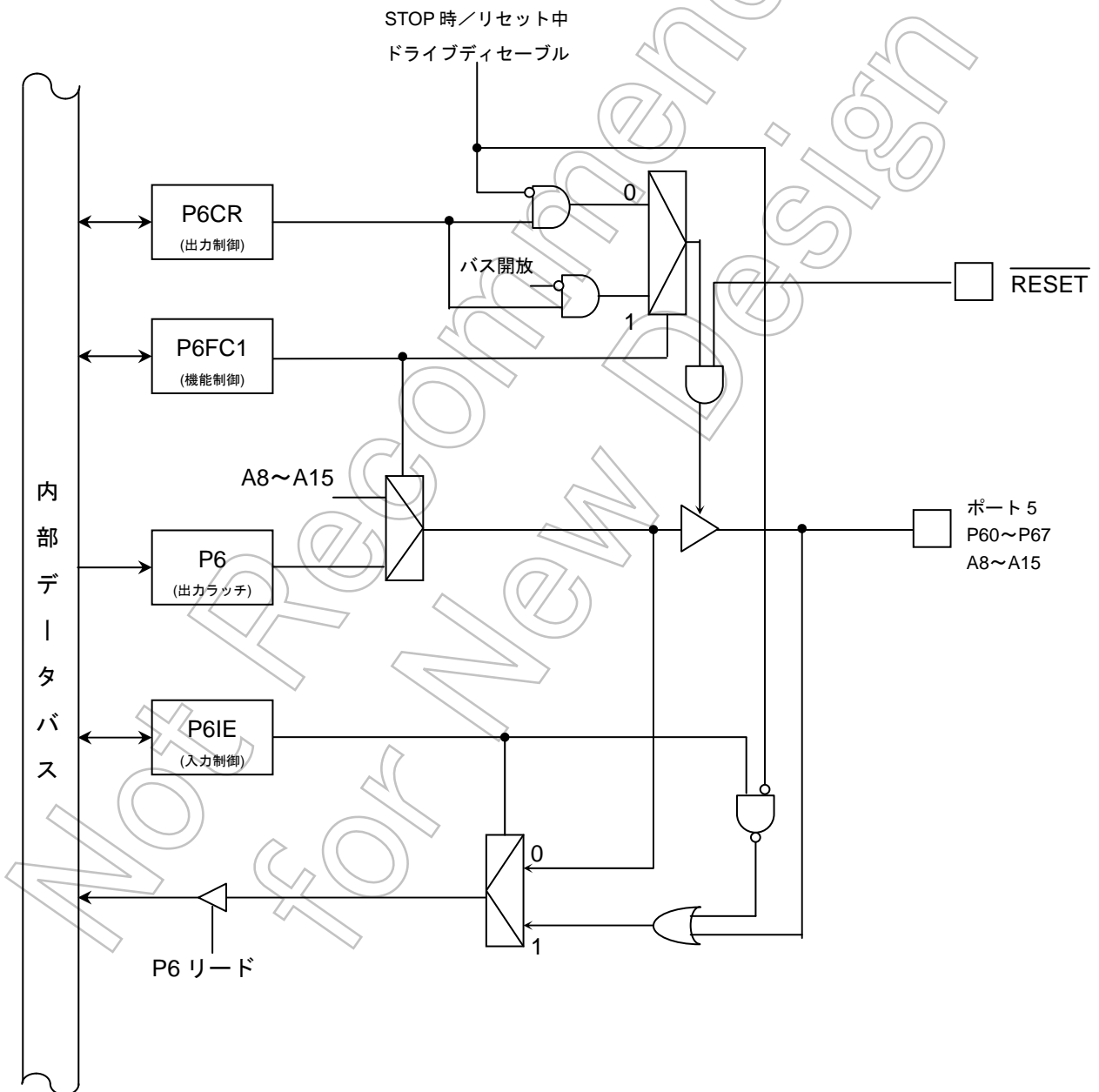
図 7-12 ポート 6 (P60~P67)
